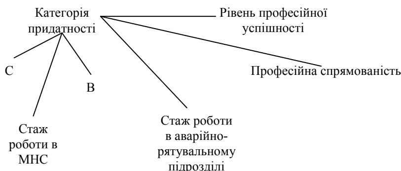
Рис. 1 – Кореляційна структура компонентів, що визначають категорію придатності фахівця аварійно-рятувального підрозділу до дій в екстремальній ситуації
