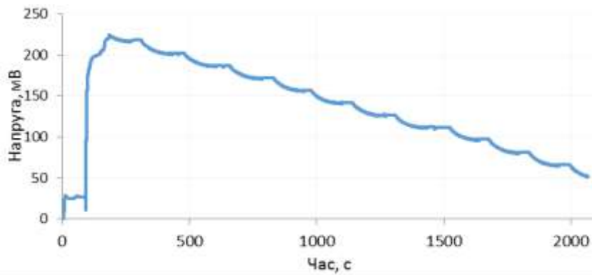
Рисунок 2 Приклад калібрувального графіка
