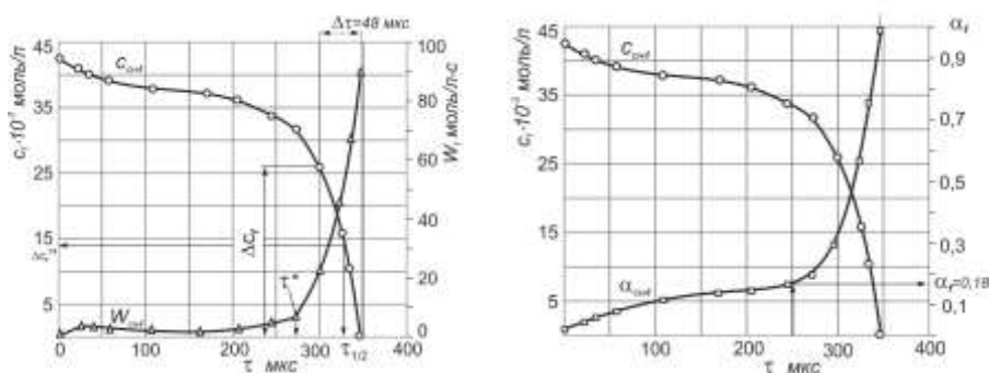
Рис. 2 – Кинетические кривые изменения концентрации метана c_f ( \circ ), скорости горения W_f ( \Delta ) и доли метана вступившего в реакцию \alpha_f ( \square ) от времени протекания реакции \tau
