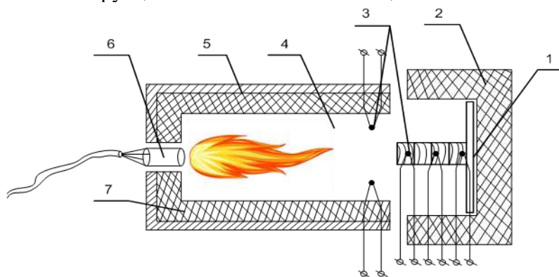
Рис.1. Експериментальна установка для вогневих випробувань зразків-фрагментів дерев'яних балок: 1 – зразок для дослідження, 2 – теплоізоляція зразка; 3 – місця установки термопар; 4 – камера теплового впливу печі; 5 – корпус печі; 6 – газовий пальник; 7 – теплоізоляція камери теплового впливу печі.
