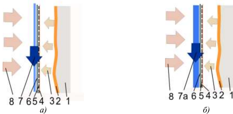
Рис.1 - Схема теплових потоків в протитепловому одязі, що має зовнішнє проточне охолодження струменями: а – водяними; б – пінними: 1 – тіло; 2 – виделення поту на шкірі; 3 – потік тепла від тіла; 4 – конденсат на тканині; 5 – вологопрониклива тканина; 6 – непрониклива оболонка; 7, 7а – відповідно водяний та пінний поверхневі струмені охолодження; 8 – зовнішній тепловий потік від пожежі
