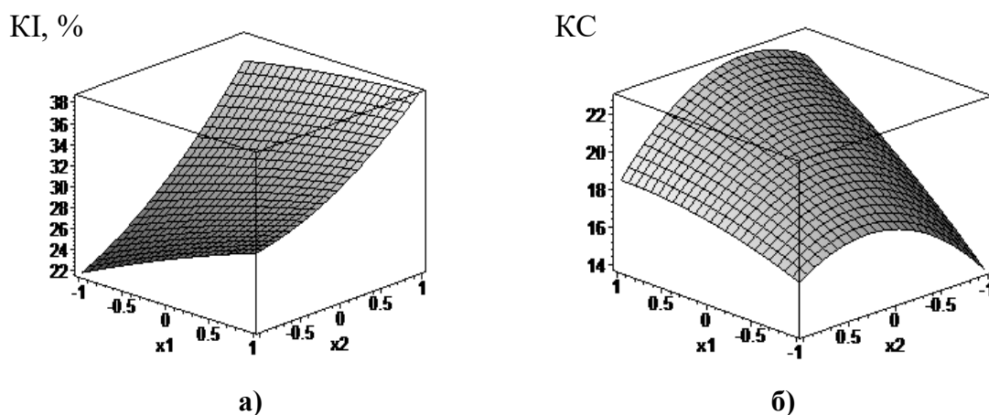
Рисунок 1 – Залежність величини кисневого індексу КІ (а) та кратності спучування КС (б) від вмісту амофосу x_1 та тригідрату оксиду алюмінію x_2
