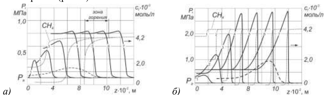
Рис. 1 – Динамика профиля давления P и концентрации метана c_f в процессе зажигания и горения газозвушной смеси в режиме дефлаграции (а) и детонации (б), вдоль оси z , для параметров макрокинетики взрывного (сплошная линия) и ламинарного горения (пунктир)
