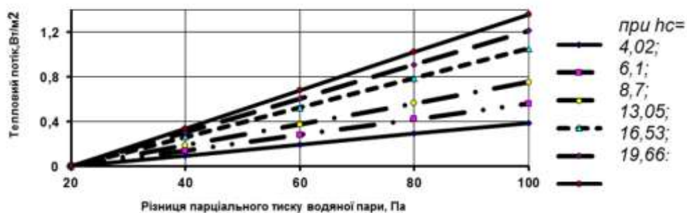
Рис. 2 - Вплив параметрів пароповітряної суміші ( P_k - P_c ) на теплової потік, що створений випаровуванням поту при температурі 50°C
