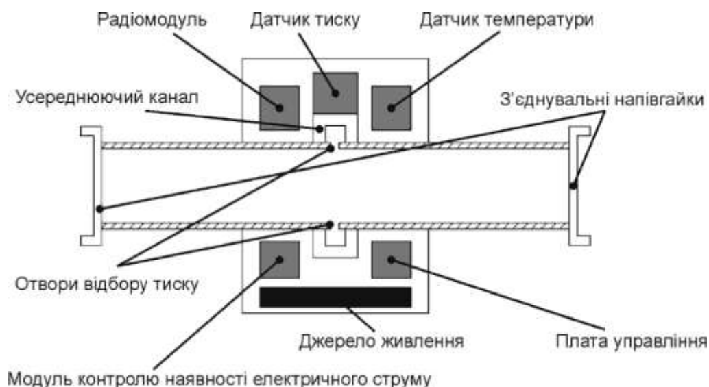
Рис. 1 - Пристрій контролю
