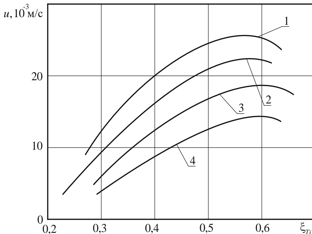
Рис. 1. Залежність швидкості горіння u нітратно-титанових сумішей від вмісту у них титану ( K_Y = 0,75 ; марка Ti – ПТМ): 1 – Ti + Sr(NO_3)_2 ; 2 – Ti + Ba(NO_3)_2 ; 3 – Ti + NaNO_3 ; 4 – Ti + KNO_3 .
