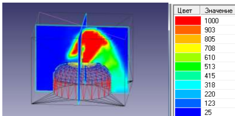
Рис. 1. Факел полум'я при пожежі у ферментаторі
