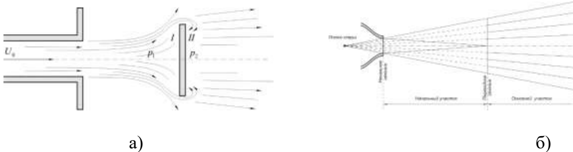
Рис.1. Приклад використання стенду а) для вивчення обтікання потоком рідини перешкоди (диска). [2]. I, II - різні зони тисків p; б) ізотакії вільної струменя, розраховані за місцевими осьовими швидкостями
