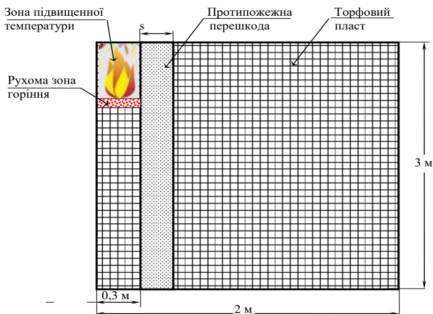
Рис. 1. Геометрична конфігурація розрахункових областей системи торфовий пласт – протипожежна перешкода
