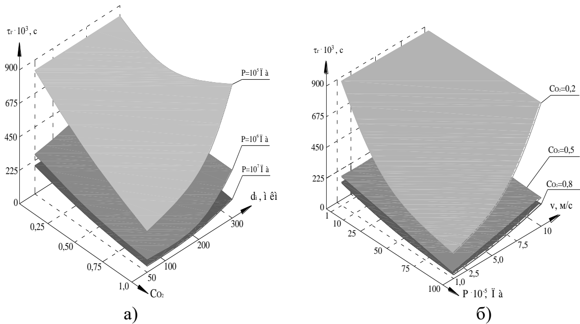
Рис. 1. Тривимірне зображення залежностей часу згорання частинки алюмінію в газовому потоці \text{O}_2 + \text{N}_2 від таких параметрів: а) – від d_m та \text{CO}_2 ( v = 1 \text{ м/с} ); б) – від v та P ( d_m = 50 \text{ мкм} ).
