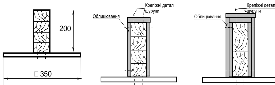
Рис. 1. Загальний вигляд експериментального зразка без вогнезахисного облицювання, з 1-м шаром та з 2-м шаром вогнезахисту.
