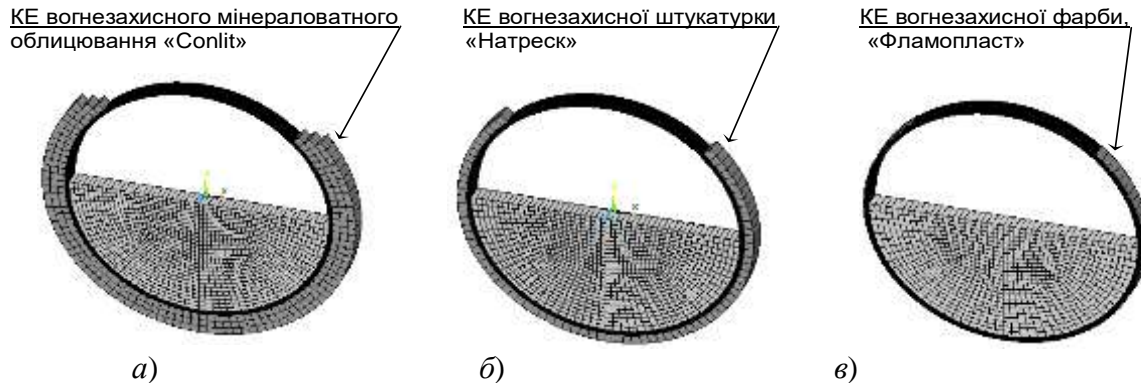
Рисунок 1. Кінцево-елементні схеми трубобетонної колони із різними вогнезахисними системами: а - «Conlit SL150»; б - «Натреск»; в - «ПІРО-СЕЙФ ФЛАМОПЛАСТ СП-А2»
