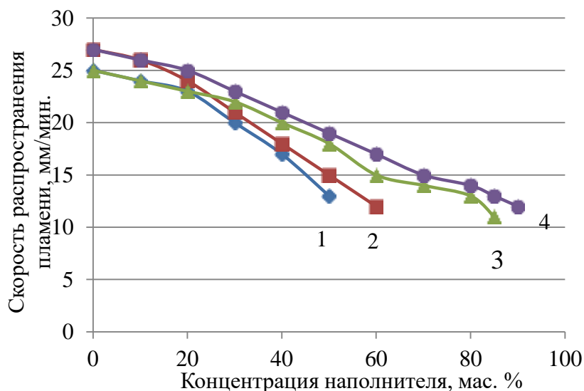
Рисунок 1. Залежність швидкості поширення пламени за стандартом UL94-НВ від концентрації Al(OH)_3 (1, 2) та Al_2O_3 (3, 4) для полістиролу (1, 3) та поліетилену (2, 4).
