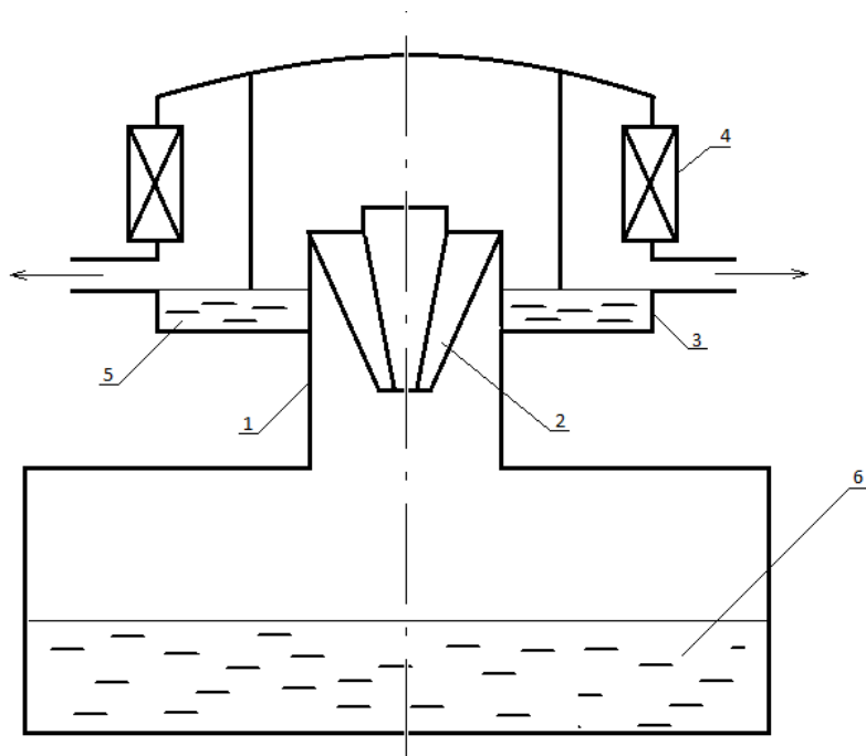
Рис. 1. Принципова технологічна схема очистки пароповітряної суміші
