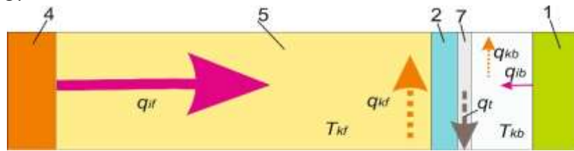
Рис. 1.3 Схема розподілу теплової енергії в системі «пожежа – ПТО – рятувальник» із проточним рухом теплоносія: q_b – потік енергії, що виносить теплоносія; 7 – канал руху теплоносія; інші позначення, як на рис. 1.2
