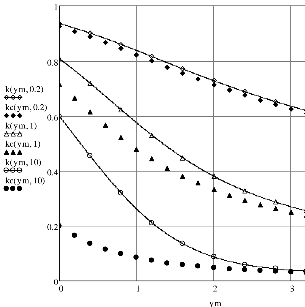
Рис. 1. Графики зависимости коэффициентов ослабления теплового потока защитным слоем случайной толщины k(ym, Bi) и соответствующим ему защитным слоем постоянной толщины kc(ym, Bi) при различных значениях критерия Bi
