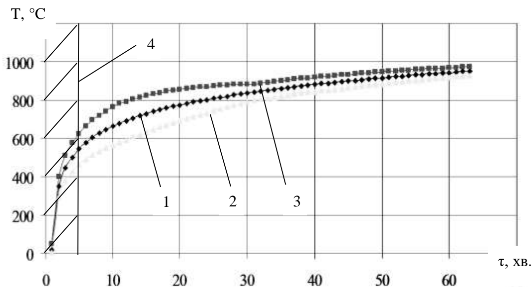
Рис. 1. Стандартний температурний режим:
