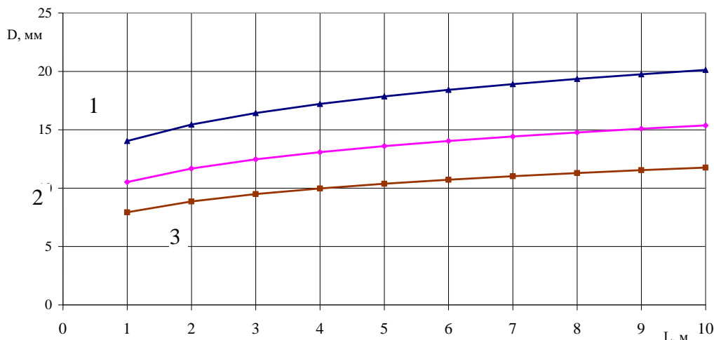
Рис.1 Залежність діаметра трубопровода від довжини участка і расхода при p=40 бар: 1 – Q=200 кг/мин; 2 – Q=100 кг/мин; 3 – Q=50 кг/мин
