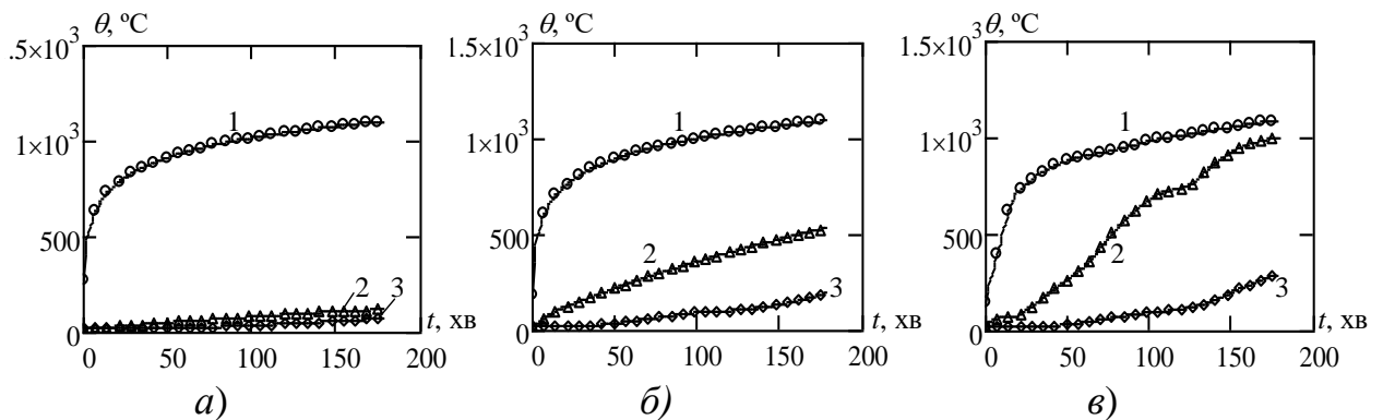
Рисунок 3 – Залежність температури поверхні колони (1), сталеві оболонки (2) та середини бетонного ядра колони (3) із різними вогнезахисними системами: а – «Conlit SL150»; б – «Натреск»; в – «ПИРО-СЕЙФ ФЛАМОПЛАСТ СП-А2» від часу
