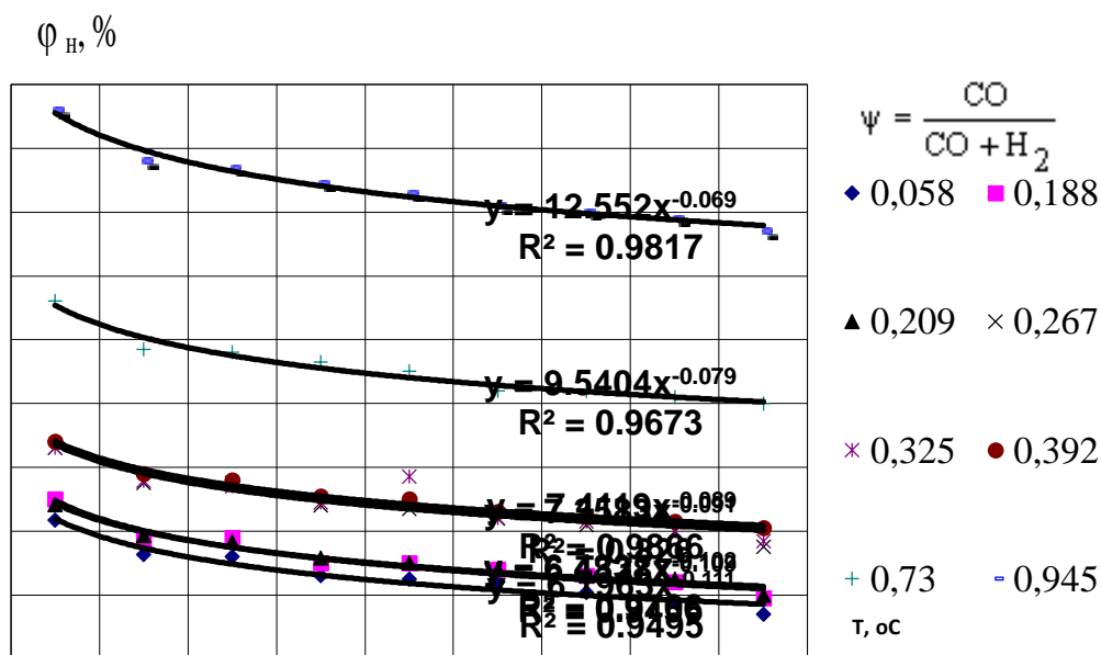
Рис. 1. Залежність нижніх КПП пламени ( \varphi_n ) від початкової температури ( T ) і складу газової суміші ( \psi ).
