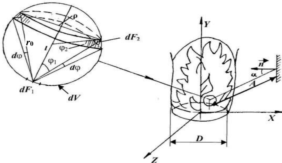
Рис. 1 Модель теплового випромінювання осередком пожежі
