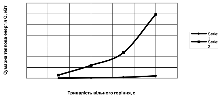
Рис. 1. Вплив тривалості вільного горіння \tau на сумарну теплову енергію: ряд 1 – v_{\Gamma} = 0,004 м/с, форма пожежі кутова 90^\circ ; ряд 2 – v_{\Gamma} = 0,016 м/с, форма пожежі кутова 180^\circ
