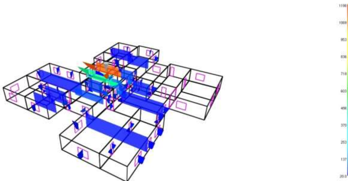
Рисунок 1 – Розвиток пожежі за допомогою моделі CFAST
