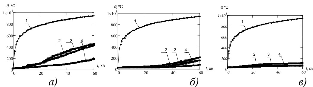
Рисунок 3 – Графіки залежності температури від часу експонування при 60 хвилинних вогневих випробувань: 1 – середнє значення температури у камері установки; 2 – середня температура у першій внутрішній контрольній точці зразка; 3 – середня температура у другій внутрішній контрольній точці зразка; 4 – середня температура у третій внутрішній контрольній точці зразка; а) зразки без вогнезахисту; б) зразки з 1-м шаром вогнезахисного облицювання OSB-3; в) зразки з 2-м шаром вогнезахисного облицювання OSB-3.
