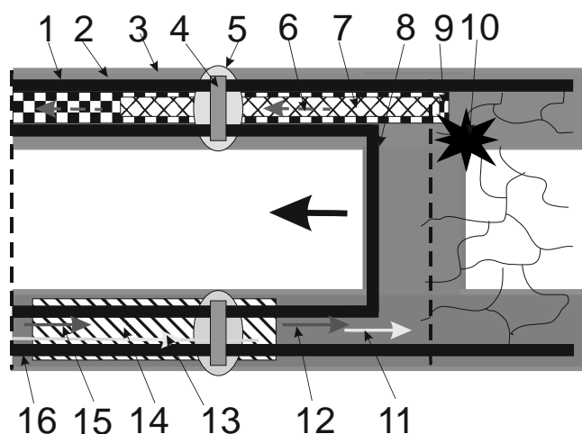
Rysunek 1 – Lokalizacja stref reagowania awaryjnego
