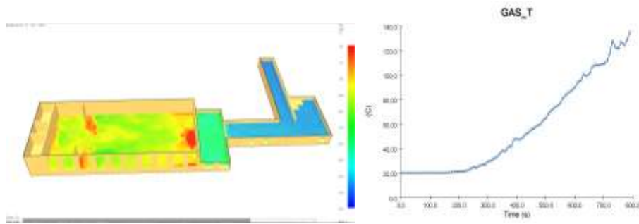
Рисунок 3 – Візуалізація результатів моделювання
