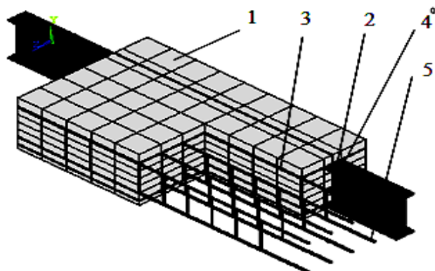
Рис. 1. Розрахункова схема горизонтальної конструкції для проведення розрахунку межі вогнестійкості (1 – КЕ бетону, 1 – КЕ сталевої двотаврової балки, 3-5 – КЕ арматури).
