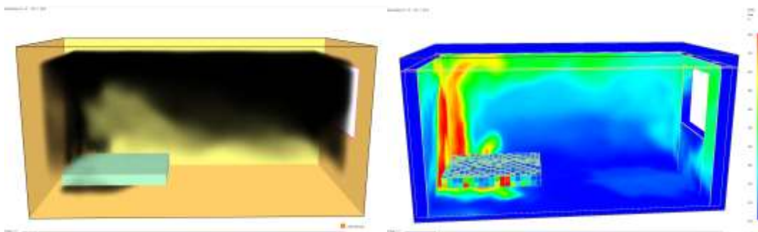
Рисунок 2 – Моделювання пожежі та візуалізація теплових полів
