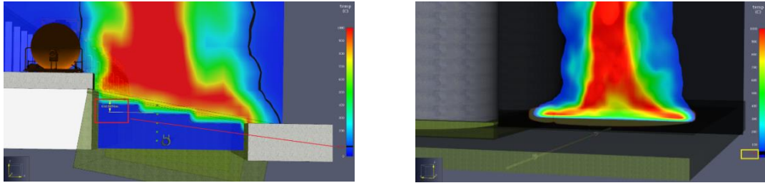
Рис. 1. Візуалізація максимальної глибини прогріву ґрунту до критичного значення: зліва – залізнична естакада, справа – нафтоцистерни
