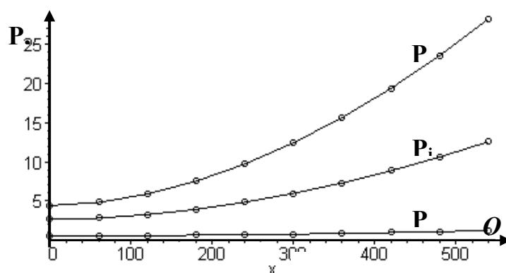
Рисунок 1 – График зависимости давления на выходе из насосной станции от расположения расчетного участка:
