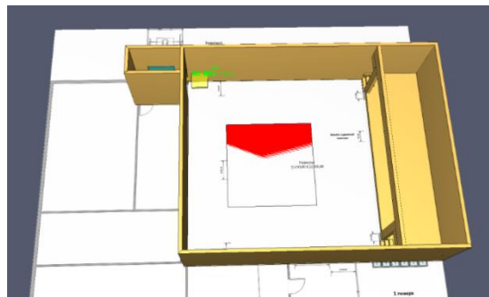
Рисунок 2 - План поверху в графічному редакторі Pyrosim
