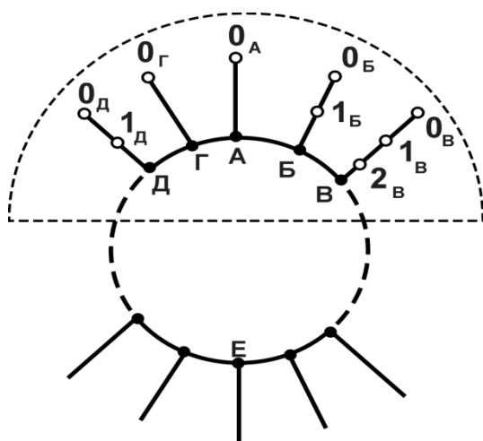
Рисунок 1 – Пример кольцевой распределительной сети
