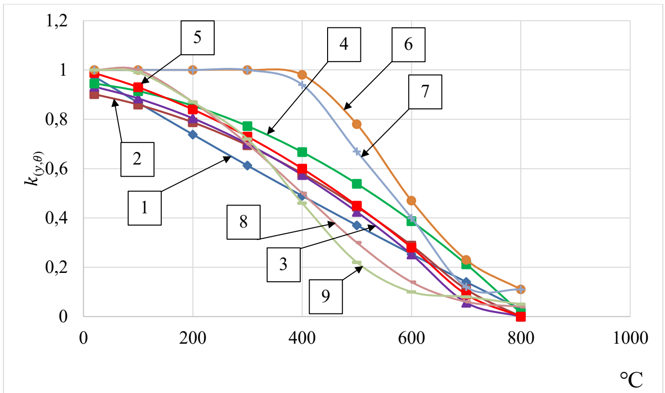
Рисунок 2.10 – Порівняльний графік значень величин коефіцієнтів зниження розрахункового опору арматури залежно від температури k_{y,\theta} :
