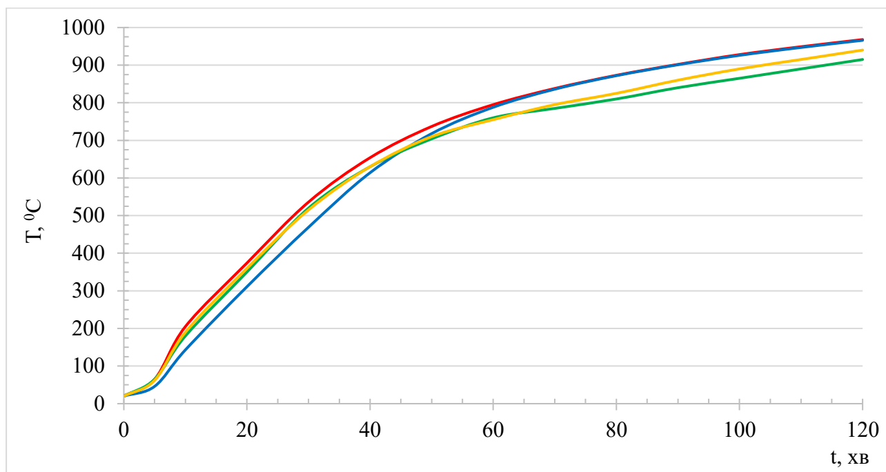
Рисунок 4.26 – Графік зміни температури бетону на глибині 1 см від поверхні конструктивних елементів за результатами чисельного моделювання: 1 – нижня грань балки (червона крива); 2 – бічна грань балки (синя крива); 3 – нижня грань переkritтя (зелена крива); 4 – колона на відстані 200 мм від переkritтя (помаранчева крива).
