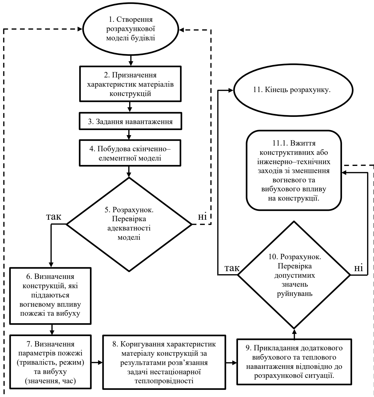
Рисунок 3.1 – Алгоритм проведення розрахунків для забезпечення стійкості монолітних залізобетонних будівель до прогресуючого обвалення внаслідок дії пожежі та дефлагарційного вибуху
