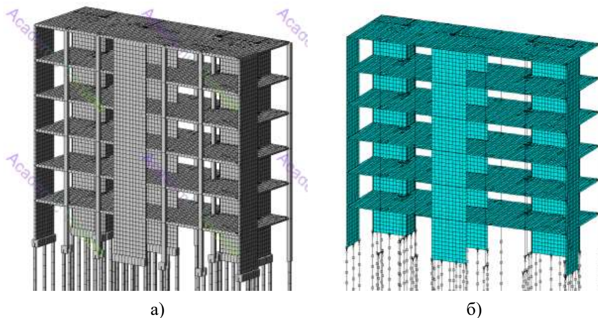
Рисунок 3.3 – Розрахункова модель: а) просторова модель будівлі; б) скінченно–елементна модель будівлі
