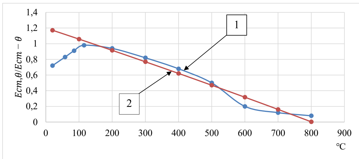
Рисунок 2.9 – Графіки залежності початково модуля пружності E_{ct,\theta}/E_{ct} - \theta від температури для важкого бетону: 1) за даними досліджень авторів; 2) за формулою 2.13
