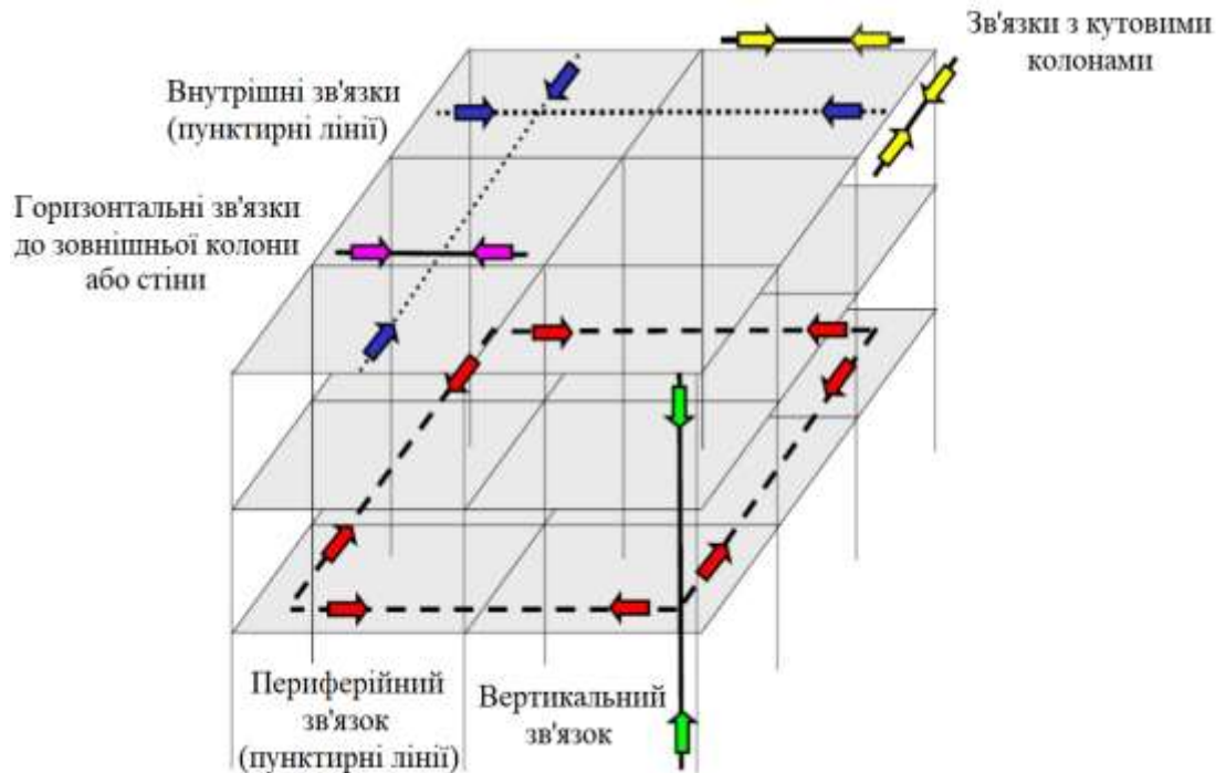
Рисунок 1.12 – Зв'язки у каркасній конструкції (UFC 4–023–03)
