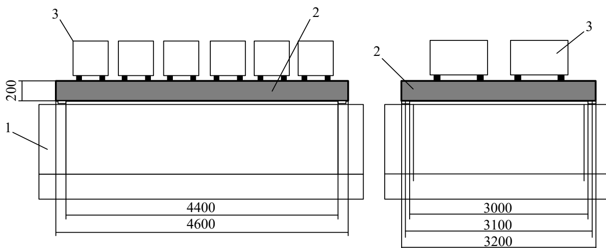
Рисунок 4.1 – Схема розташування зразків на печі: 1 – вогнева піч; 2 – плита; 3 – вантажні блоки
