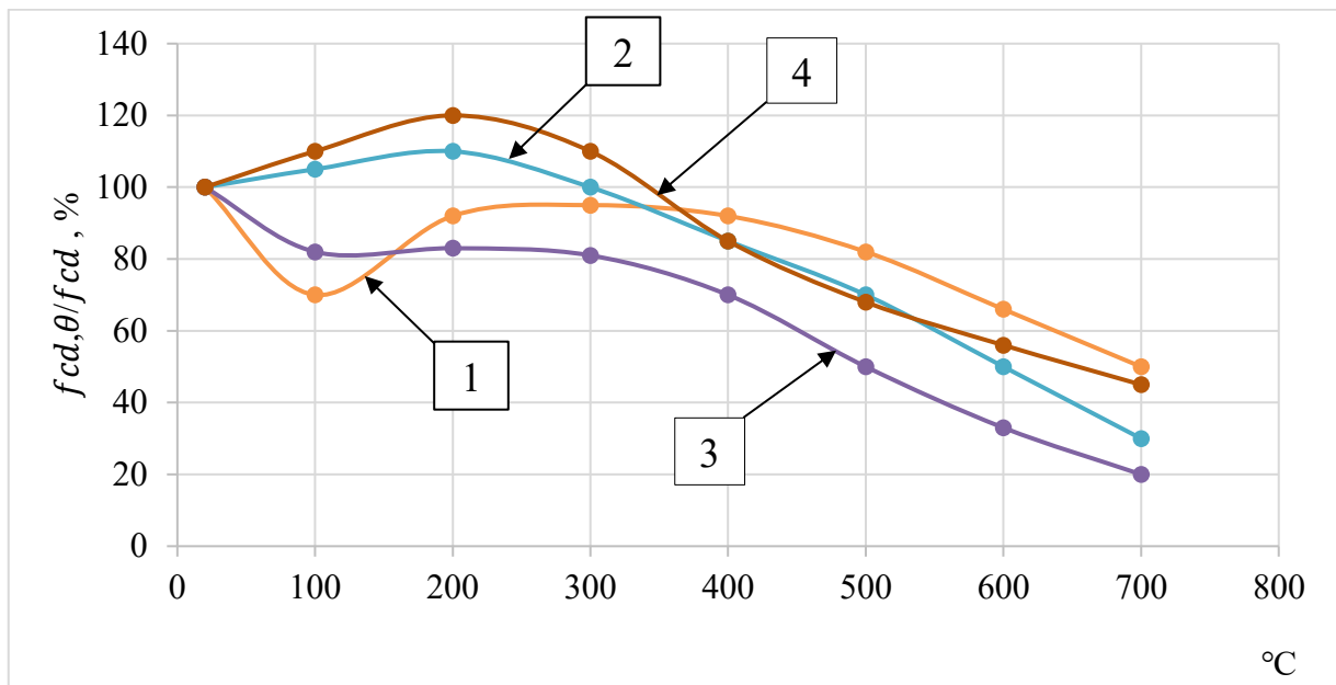
Рисунок 2.4 – Вплив високих температур на величину розрахункового значення міцності бетону на стиск: 1) звичайний важкий бетон; 2) керамзитобетон; 3) високоміцний бетон; 4) керамзитоперлітобетон
