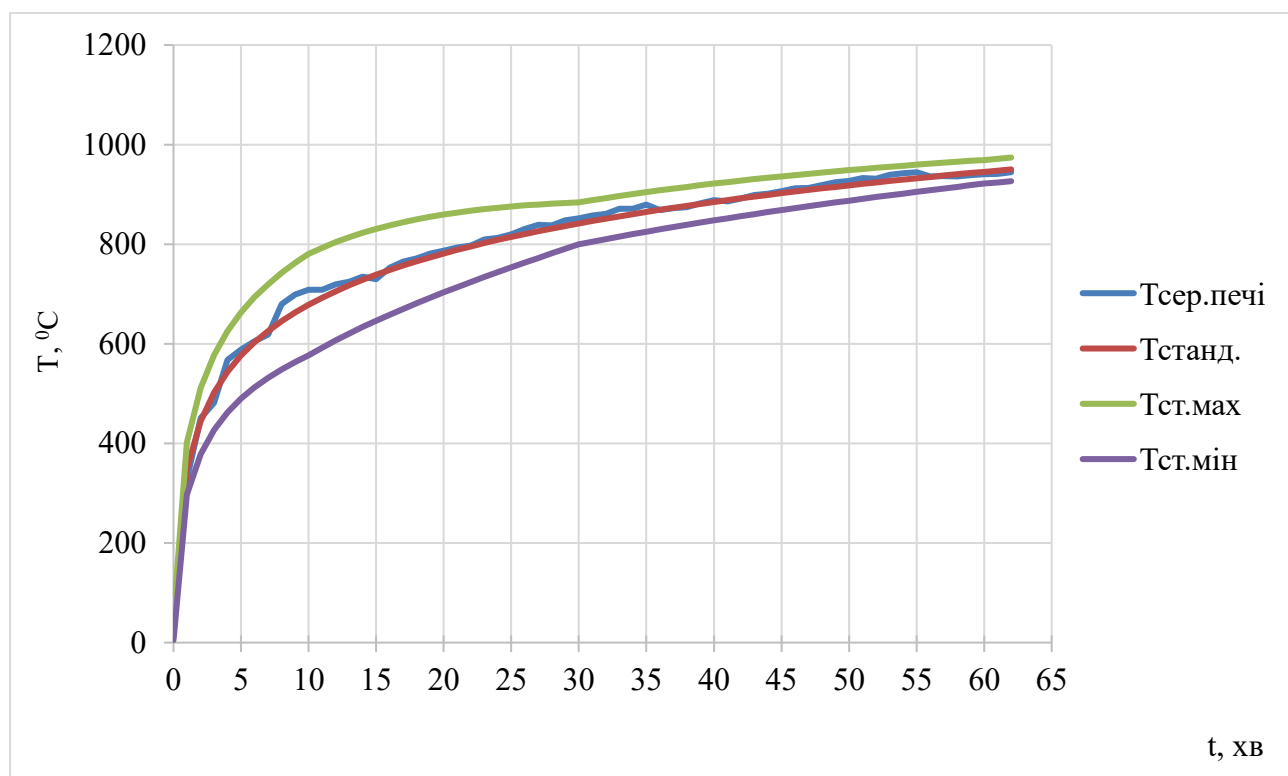
Рисунок 4.3 – Температура в печі при випробуванні зразків
