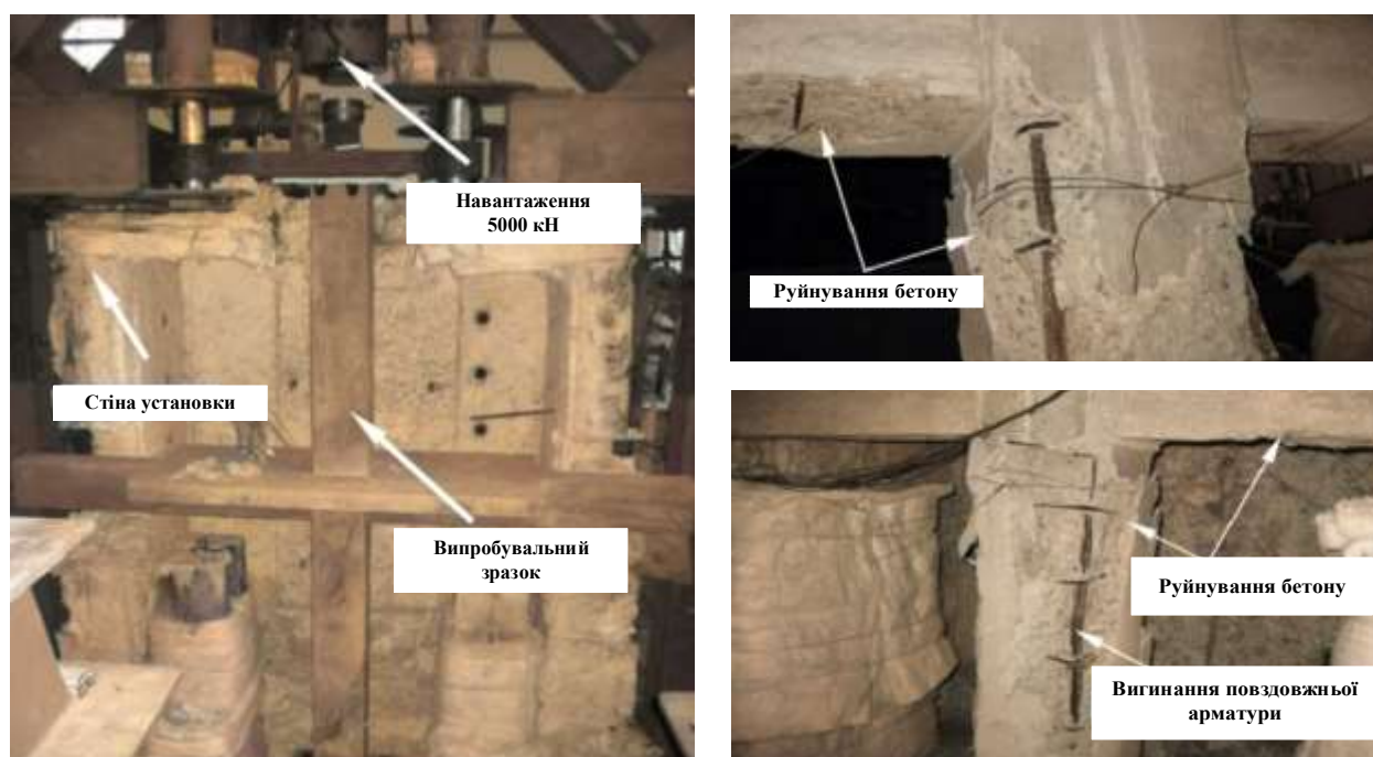
Рисунок 4.20 – Схема установки та результати випробувань [91]
