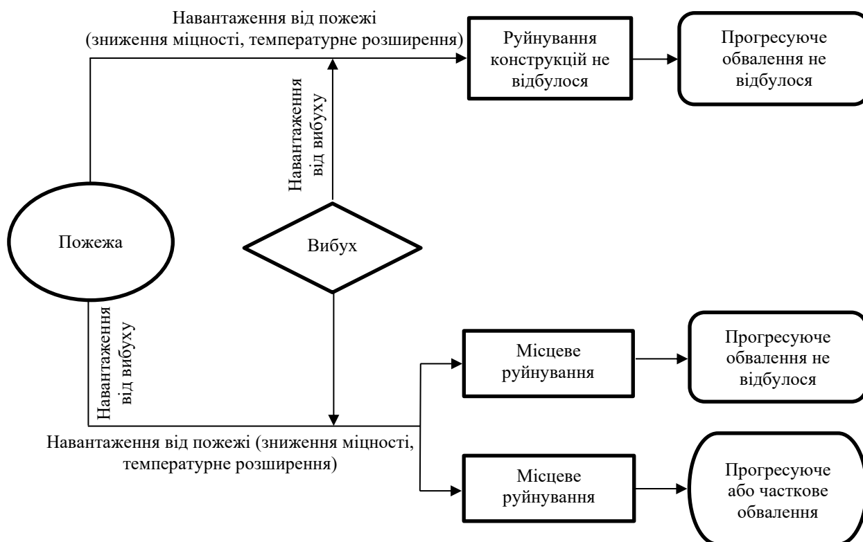
Рисунок 1.14 – Схематичне зображення механізму прогресуючого обвалення будівель внаслідок пожежі та вибуху
