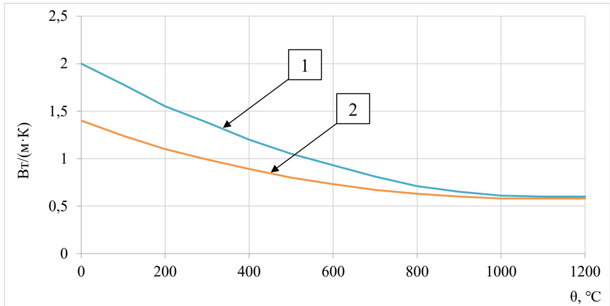
Рисунок 2.2 – Залежність теплопровідності бетону \lambda_c від температури:
