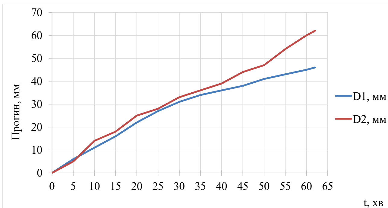
Рисунок 4.5 – Прогин випробувальних зразків
