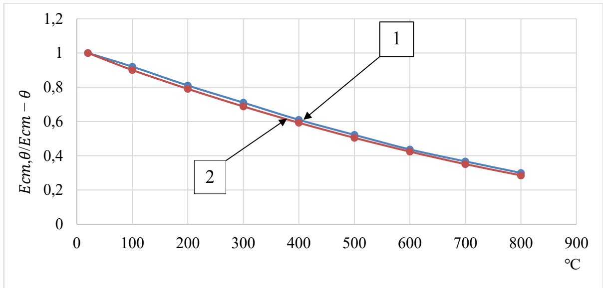
Рисунок 2.8 – Графіки залежності початково модуля пружності E_{ct,\theta}/E_{ct} - \theta від температури для керамзитобетону: 1) за даними досліджень авторів; 2) за формулою 2.12
