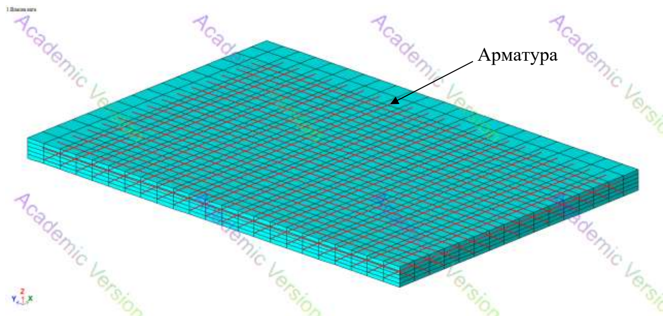
Рисунок 4.14 – Об'ємна скінченно-елементна модель плити
