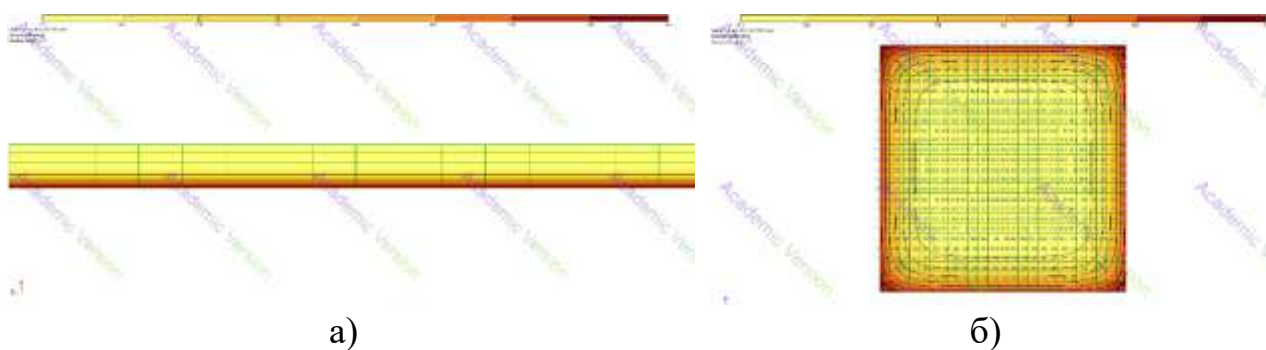
Рисунок 3.6 – Розподіл температурних полів у залізобетонних конструкціях:
