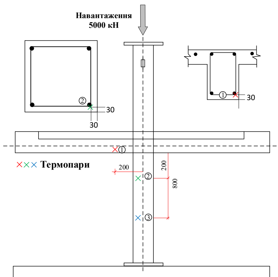
Рисунок 4.21 – Схема установки та розміщення термопар [91]
