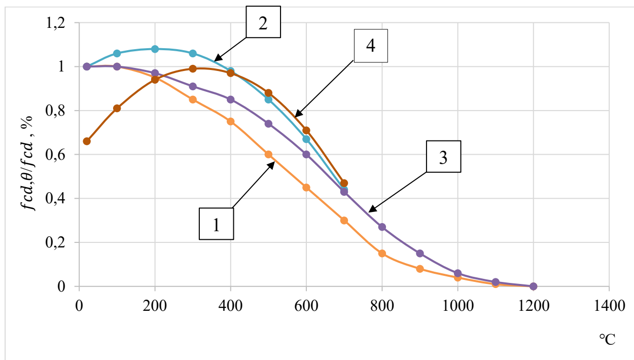
Рисунок 2.3 – Порівняльний графік зменшення міцності бетону при підвищенні температури: 1) керамзитобетон за EN 1992–1–2; 2) керамзитобетон за результатами натурних випробувань; 3) важкий бетон за EN 1992–1–2; 4) важкий бетон за результатами натурних випробувань
