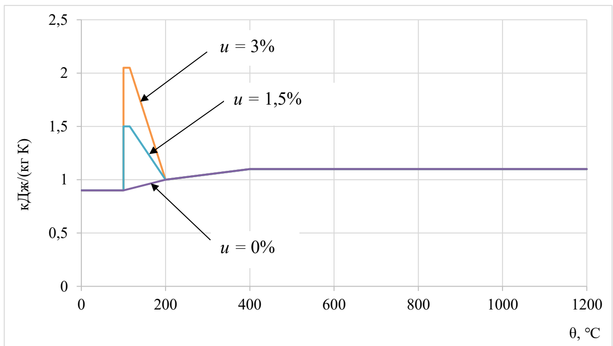
Рисунок 2.1 – Залежність питомої теплоємності c_p(\theta) бетону на силікатному заповнювачі з вологістю u = 0; 1,5 і 3\% від температури
