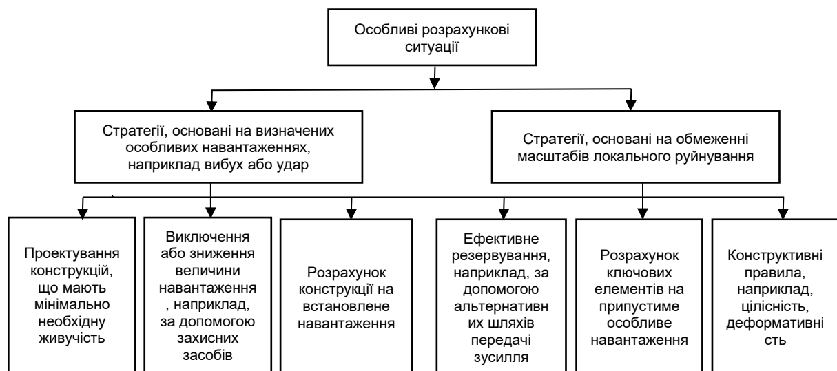
Рисунок 1.13 – Стратегії для особливих розрахункових ситуацій
