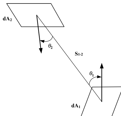
Рисунок 2.15 – Геометрична модель радіаційного теплообміну між двома диференціальними поверхнями dA_1 і dA_2 , які використовуються для розрахунку коефіцієнта форми F_{1-2}
