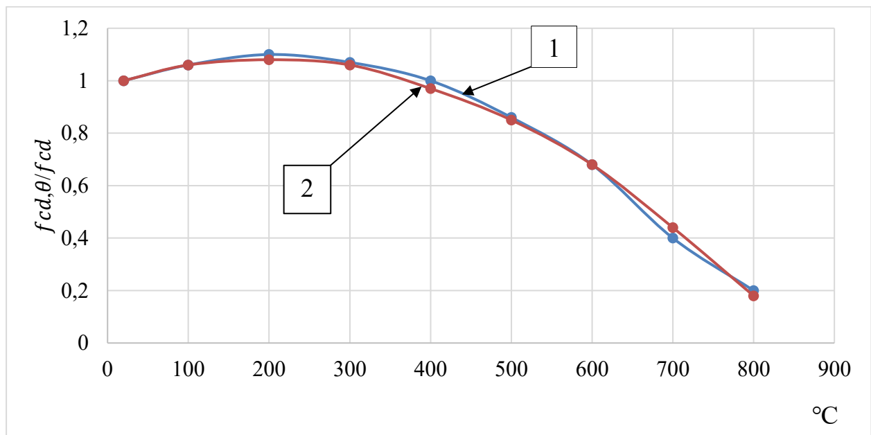
Рисунок 2.6 – Графіки залежності « f_{cd,\theta}/f_{cd} - \theta » для керамзитобетону:
