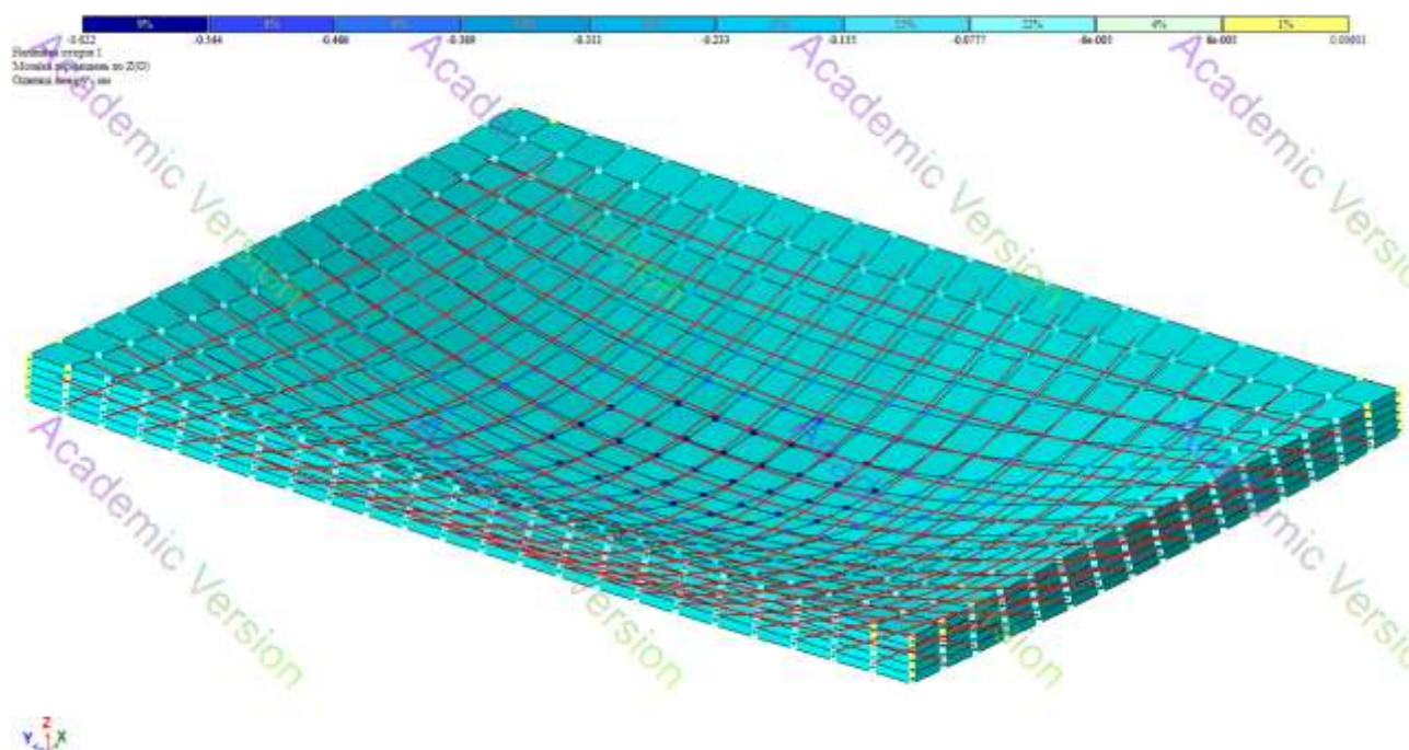
Рисунок 4.16 – Мозаїка прогинів об’ємної скінченно–елементної моделі монолітної залізобетонної плити за результатами комп’ютерного моделювання
