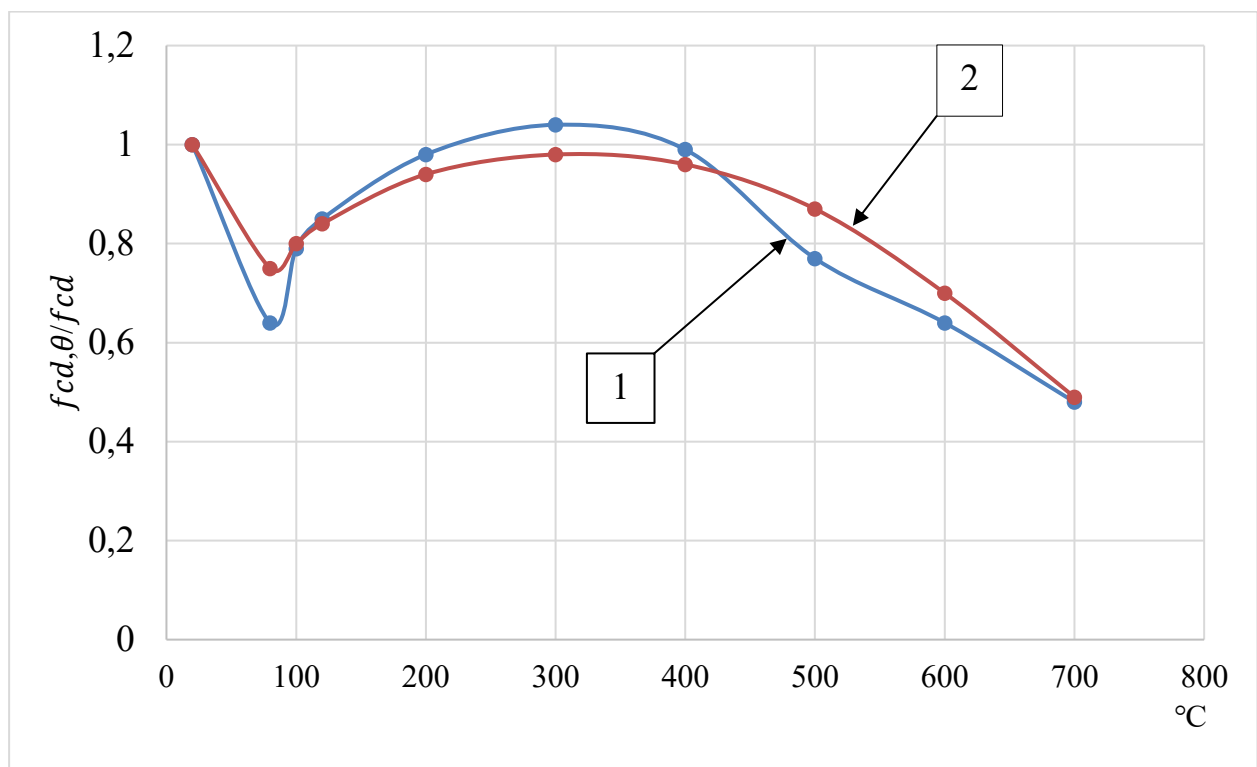
Рисунок 2.7 – Графіки залежності модуля пружності f_{cd,\theta}/f_{cd} - \theta від температури для важкого бетону: 1) характеристичні; 2) експериментальні
