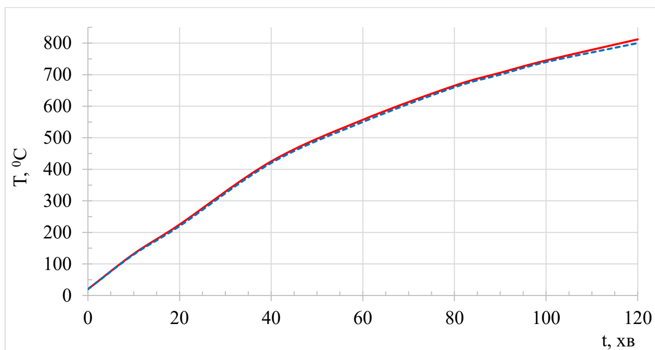
Рисунок 4.27 – Порівняння температурних значень, виміряних термопарами під час випробування (червона лінія) та у чисельному експерименті (синя лінія) в залізобетонній колоні на відстані 800 мм від балки
