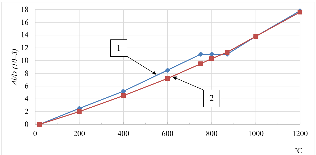
Рисунок 2.12 – Повне температурне видовження арматури: 1) ненапружена арматура; 2) попередньо напружена арматура
