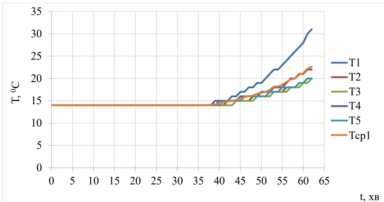
Рисунок 4.4 – Графіки середніх температур на поверхні зразків
