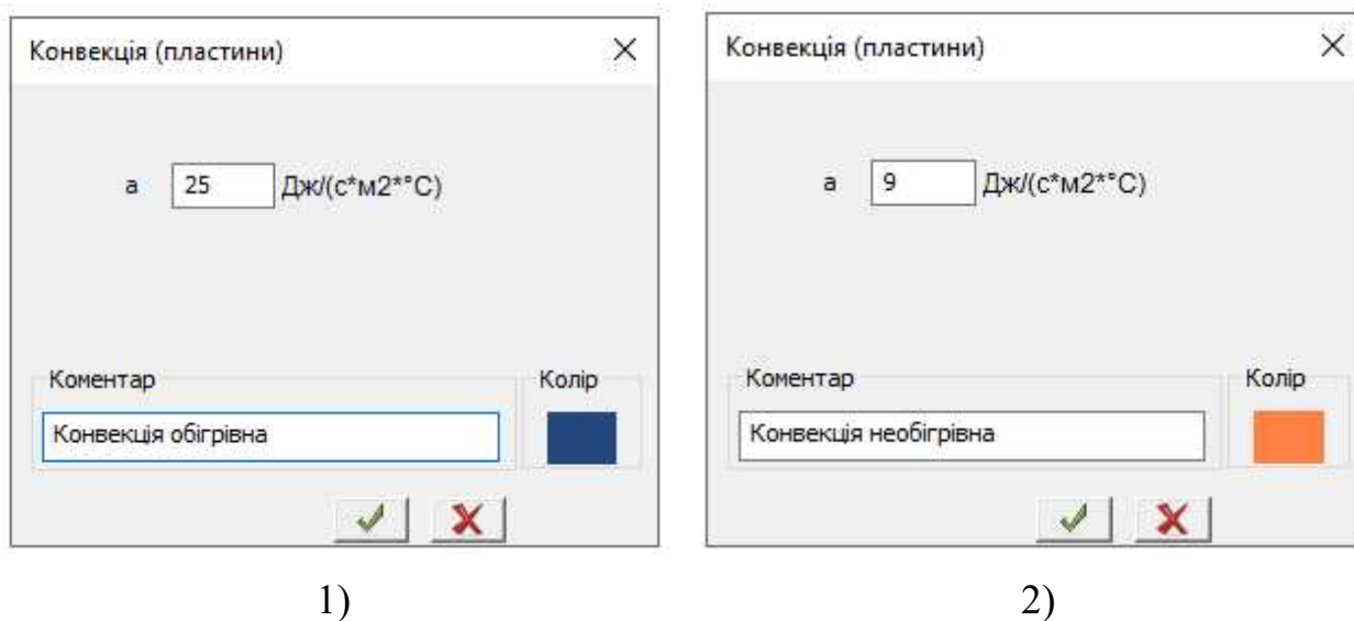
Рисунок 4.8 – Призначення коефіцієнта конвекційного теплообміну:
