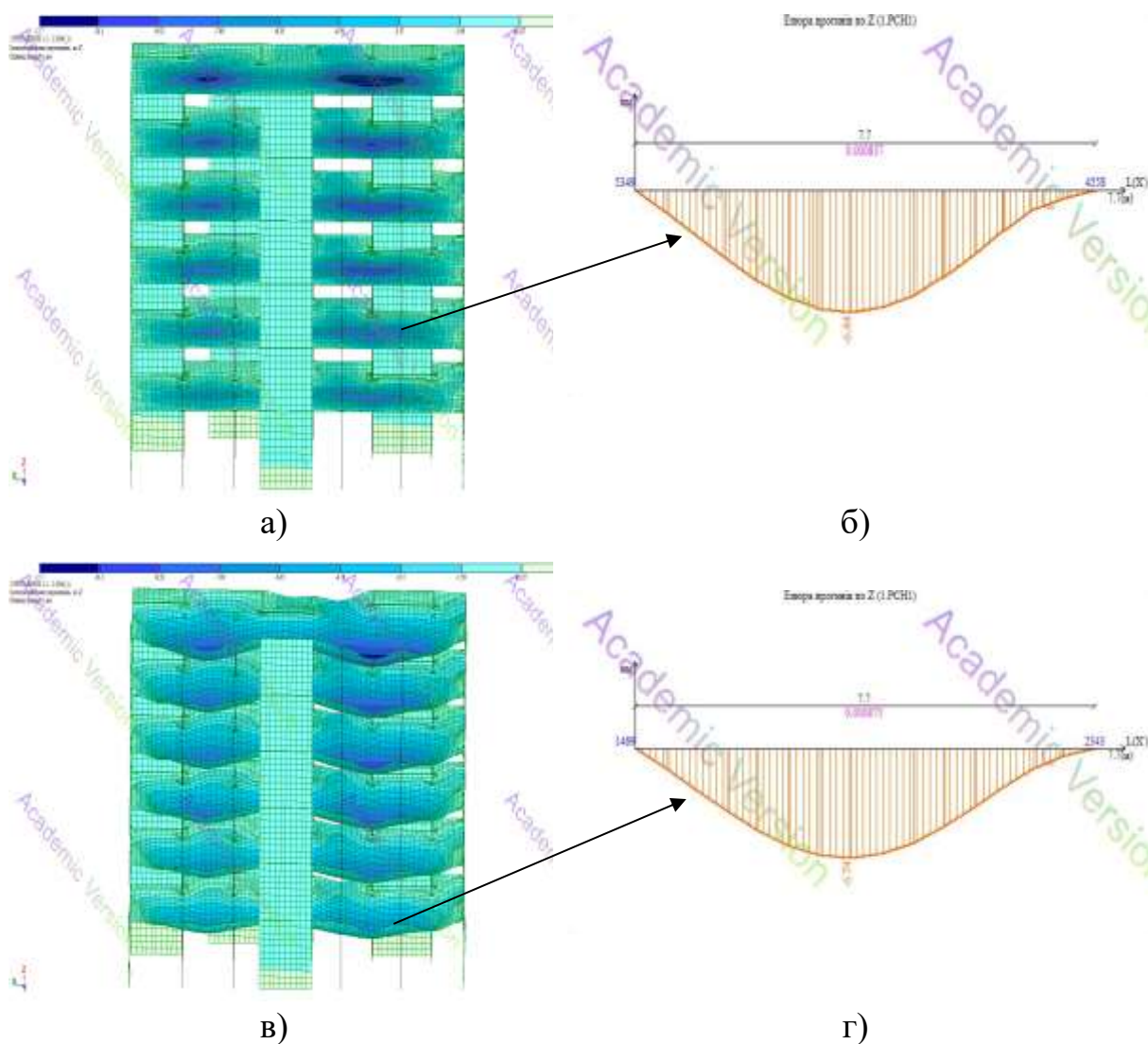
Рисунок 3.4 – Напружено-деформований стан конструкцій та переміщення до аварійних ситуацій: а) – ізополя відносних переміщень по Z; б) – епюра прогинів верхньої плити перекриття (6,44 мм); в) – ізополя переміщень по Z збільшені у 20 разів; г) – епюра прогинів нижньої плити перекриття (6,74 мм)
