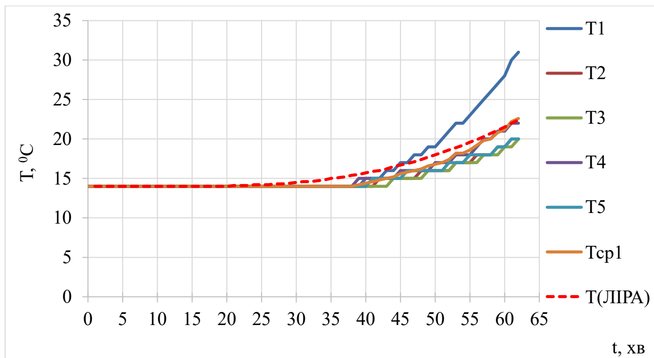
Рисунок 4.13 – Порівняльні графіки середніх температур на поверхні за результатами випробувань та комп'ютерного моделювання
