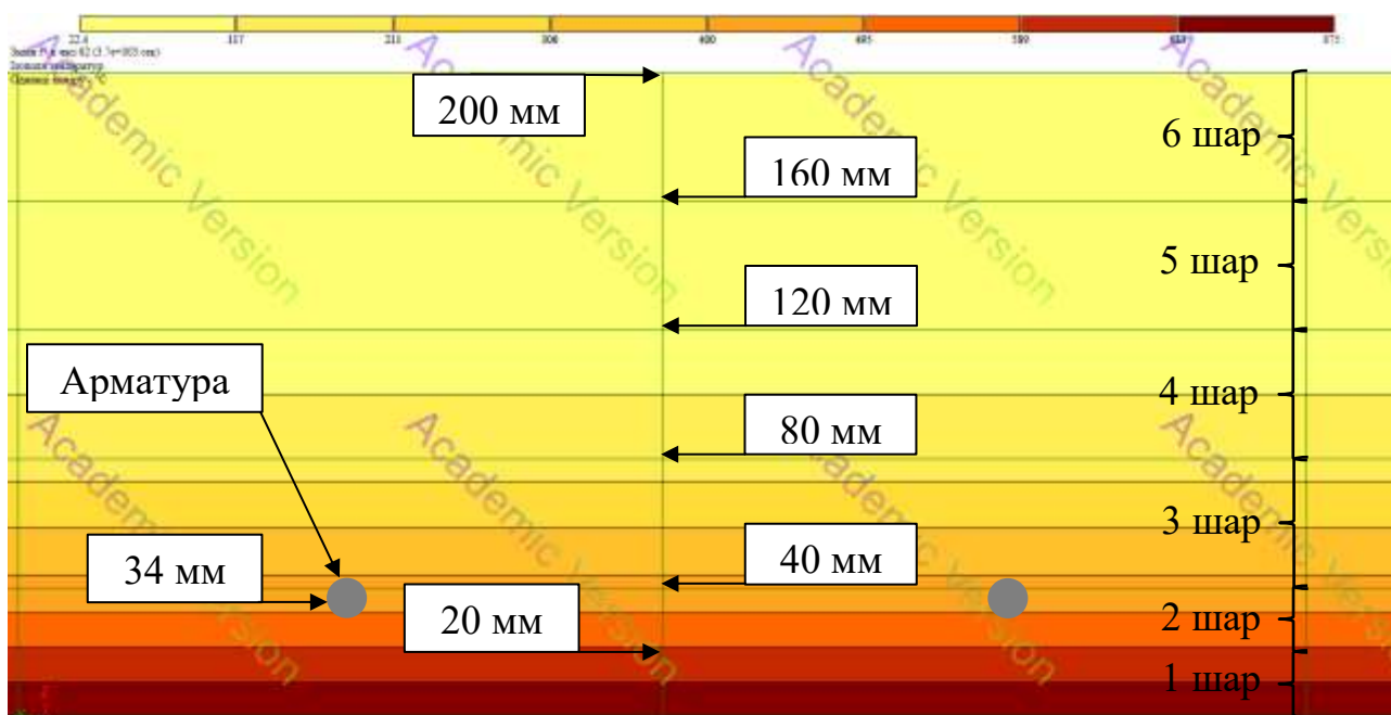
Рисунок 4.15 – Графічне зображення розподілу температурних полів в конструкції на 62 хвилині
