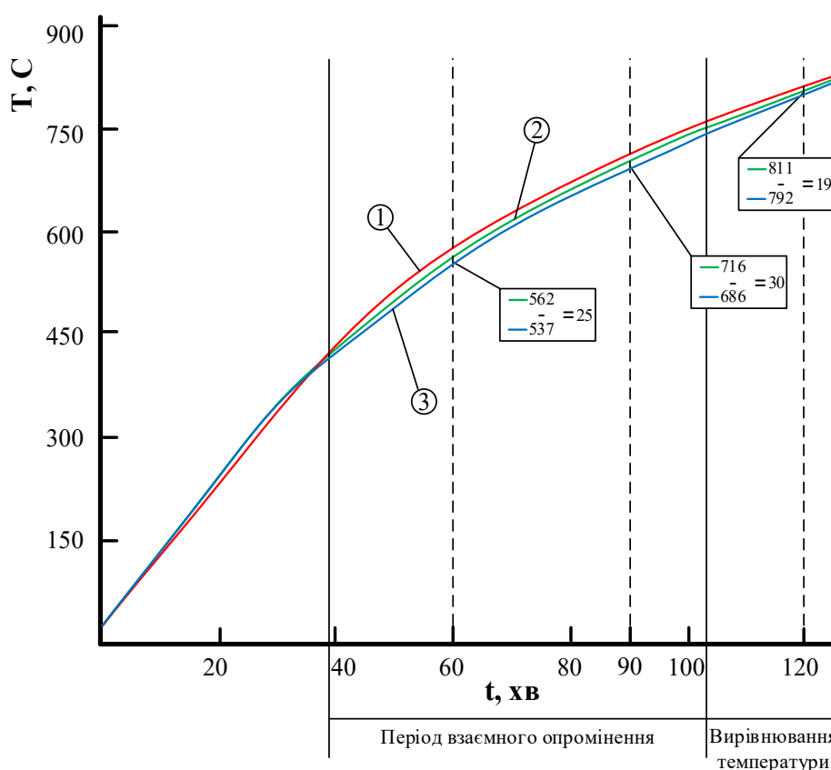
Рисунок 4.22 – Графіки різниці значень температури шару бетону на глибині 30 мм на різних відрізках часу у відповідних зонах: червона лінія – зона ділянки балки на відстані 200 мм від колони; зелена лінія – зона ділянки колони на
