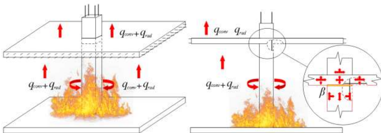
Рисунок 2.13 – Схематичне зображення механізмів теплопередачі в зоні вузла «залізобетонна колона–перекриття» під час пожежі з урахуванням конвективного, радіаційного впливу та контактного теплообміну, формалізованого через коефіцієнт \beta
