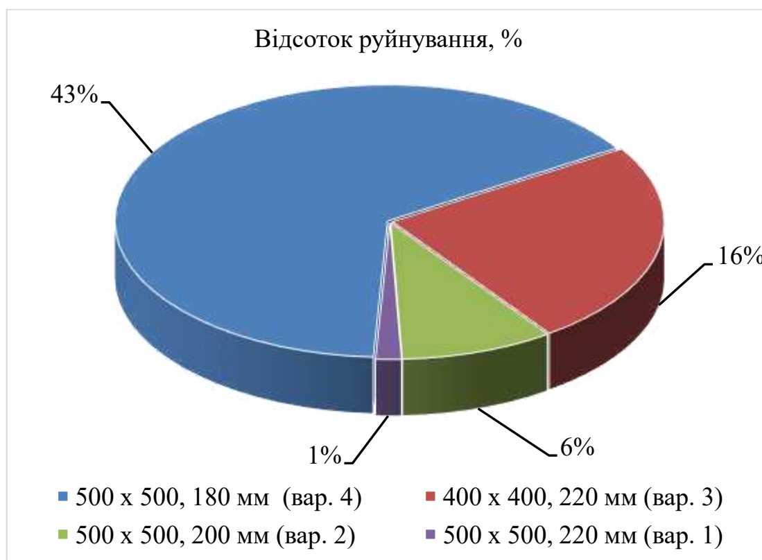
Рисунок 4.30 – Розподіл відсотка руйнування будівлі за варіантами перерізів несучих конструкцій
