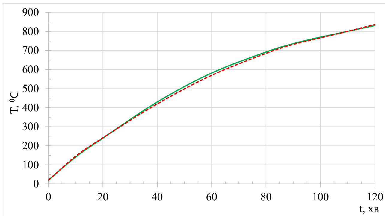
Рисунок 4.29 – Порівняння температурних значень, виміряних термопарами під час випробування (зелені лінії) та у чисельному експерименті (червоні лінії) на глибині 30 мм залізобетонної колони з урахуванням взаємного опромінення
