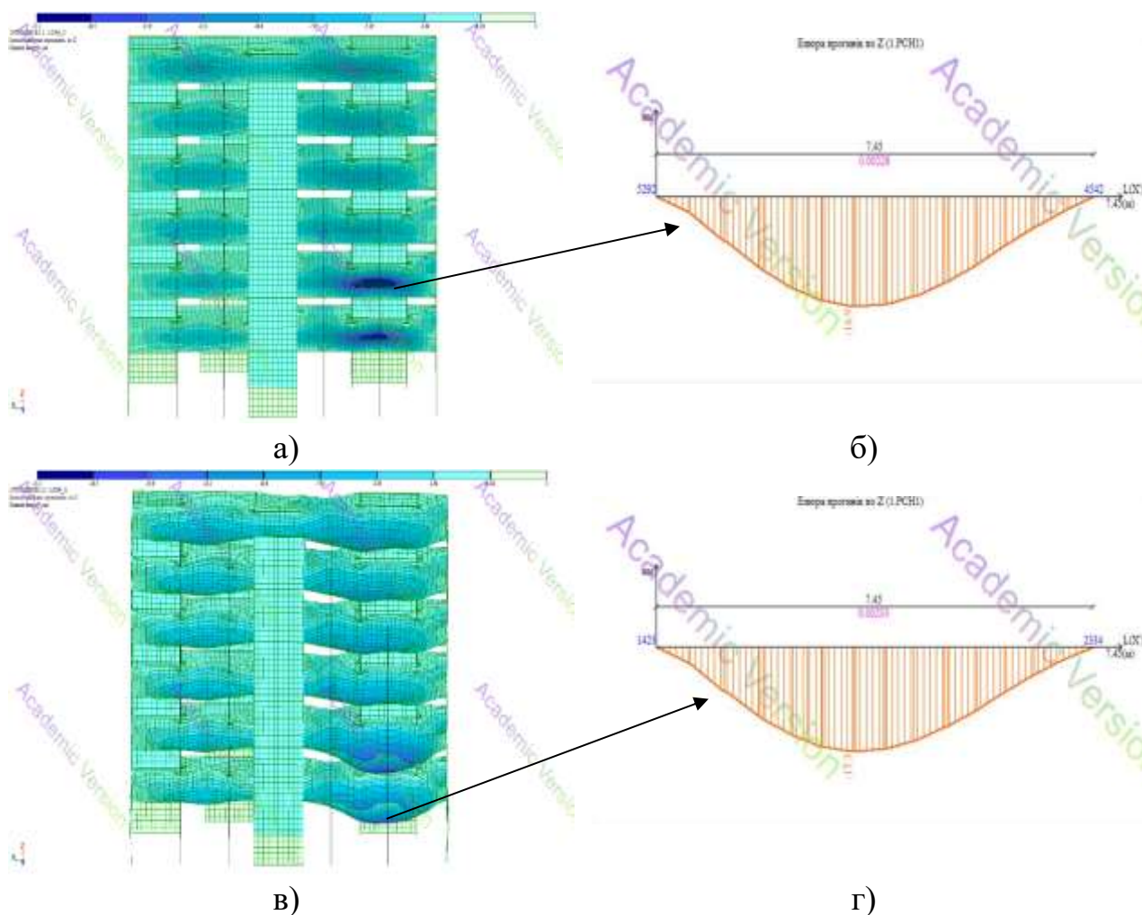
Рисунок 3.8 – Напружено–деформований стан конструкцій та переміщення при пожежі тривалістю 60 хв.: а) – ізополя відносних переміщень по Z; б) – епюра прогинів верхньої плити перекриття (16,9 мм); в) – ізополя переміщень по Z збільшені у 20 разів; г) – епюра прогинів нижньої плити перекриття (17,3 мм)
