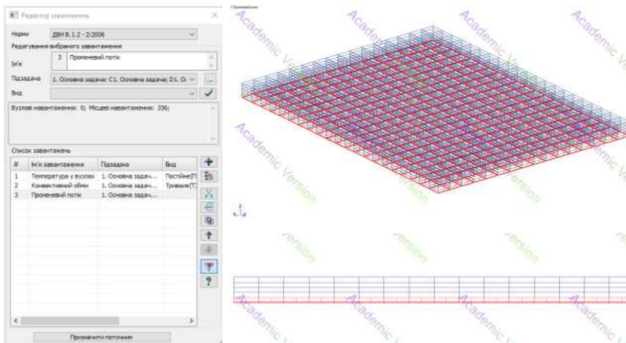
Рисунок 4.10 – Формування динамічного температурного завантаження для стержнів нижньої частини конструкції
