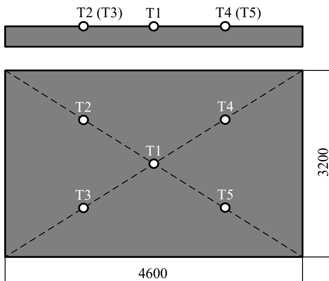
Рисунок 4.2 – Розташування термопар для вимірювань температури на необігрівній поверхні
