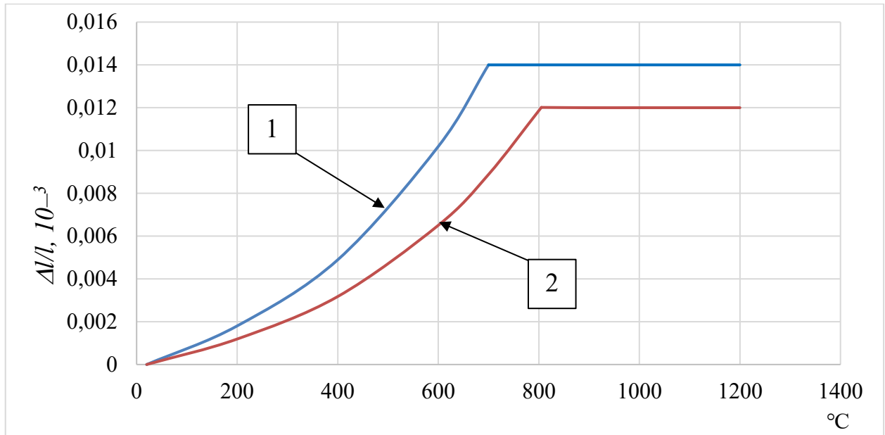
Рисунок 2.11 – Графік залежності температурного розширення від температури: 1) силікатний заповнювач; 2) карбонатний заповнювач
