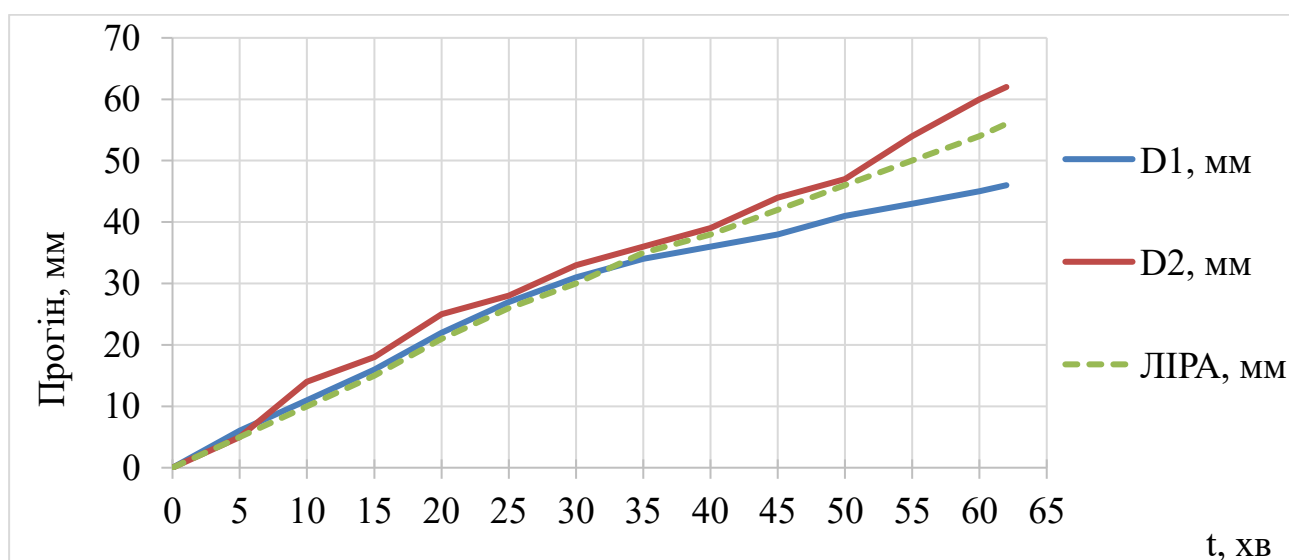
Рисунок 4.19 – Порівняльні графіки прогинів за результатами експерименту та комп’ютерного моделювання
