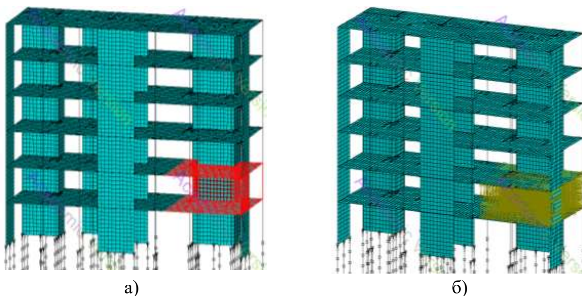
Рисунок 3.5 – Місця дії аварійного навантаження в скінченно–елементної моделі будівлі: а) – ділянка пожежі; б) – зона вибухового навантаження.
