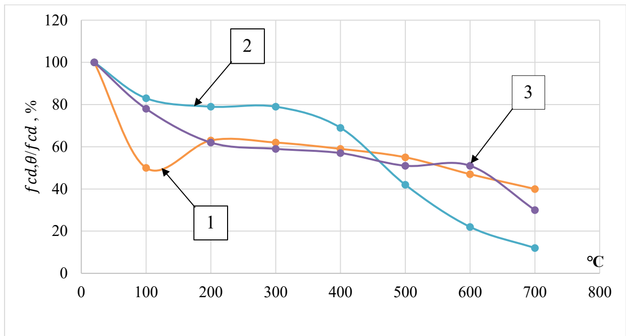
Рисунок 2.5 – Вплив високих температур на величину розрахункового значення міцності бетонів на розтяг: 1) важкий бетон; 2) високоміцний бетон; 3) керамзитоперлітобетон
