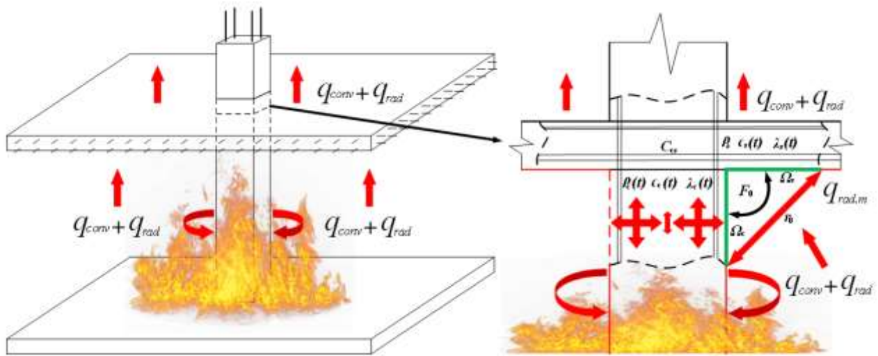
Рисунок 2.14 – Схематичне представлення моделі теплопереносу у вузлі «колона–перекриття» з урахуванням взаємного інфрачервоного випромінювання між внутрішніми поверхнями конструкцій при пожежі
