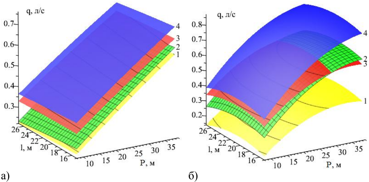
Рис. 2.6. Залежність витрат води q (л/с) від довжини рукава l (м) та тиску в мережі P (м) у разі підключення до ГПВ рукава діаметром 19 мм: 1 – s=32\% , d=6 мм; 2 – s=88\% , d=6 мм; 3 – s=32\% , d=12 мм; 4 – s=88\% , d=12 мм. а) ПЗР; б) НЖР
