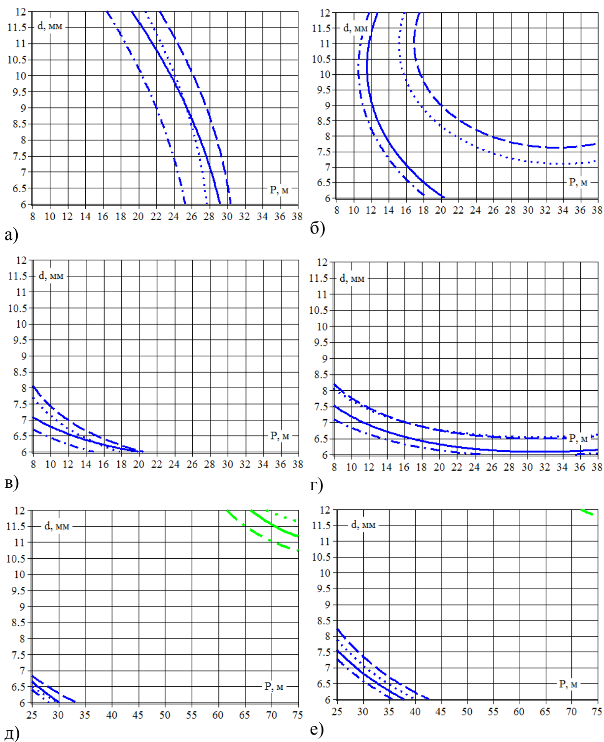
Рис. 4.7. Номограми для визначення припустимих параметрів ПКК: а) ГПВ ПЗР 19 мм; б) ГПВ НЖР 19 мм; в) ГПВ ПЗР 25 мм; г) ГПВ НЖР 25 мм; д) ВПВ ПЗР 25 мм; е) ВПВ НЖР 25 мм (див. легенду до рис. 4.8)
