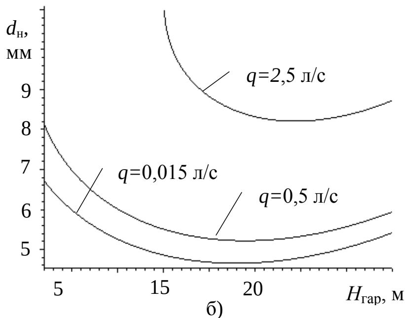
Рис. 4.6. Залежність діаметра насадка розпорошувача d_n для ПКК, приєднаного до господарсько-питної мережі, від гарантованого напору в мережі H_{гар} , укомплектованого напівжорстким рукавом діаметром: а) 25 мм; б) 33мм
