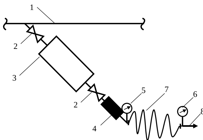
Рис. 2.1. Схема установки для експериментального дослідження фактичних витрат води з ПКК: 1 – водопровідна мережа; 2 – засувка; 3 – насос; 4 – лічильник води; 5, 6 – манометри; 7 – рукав; 8 – розпорошувач
