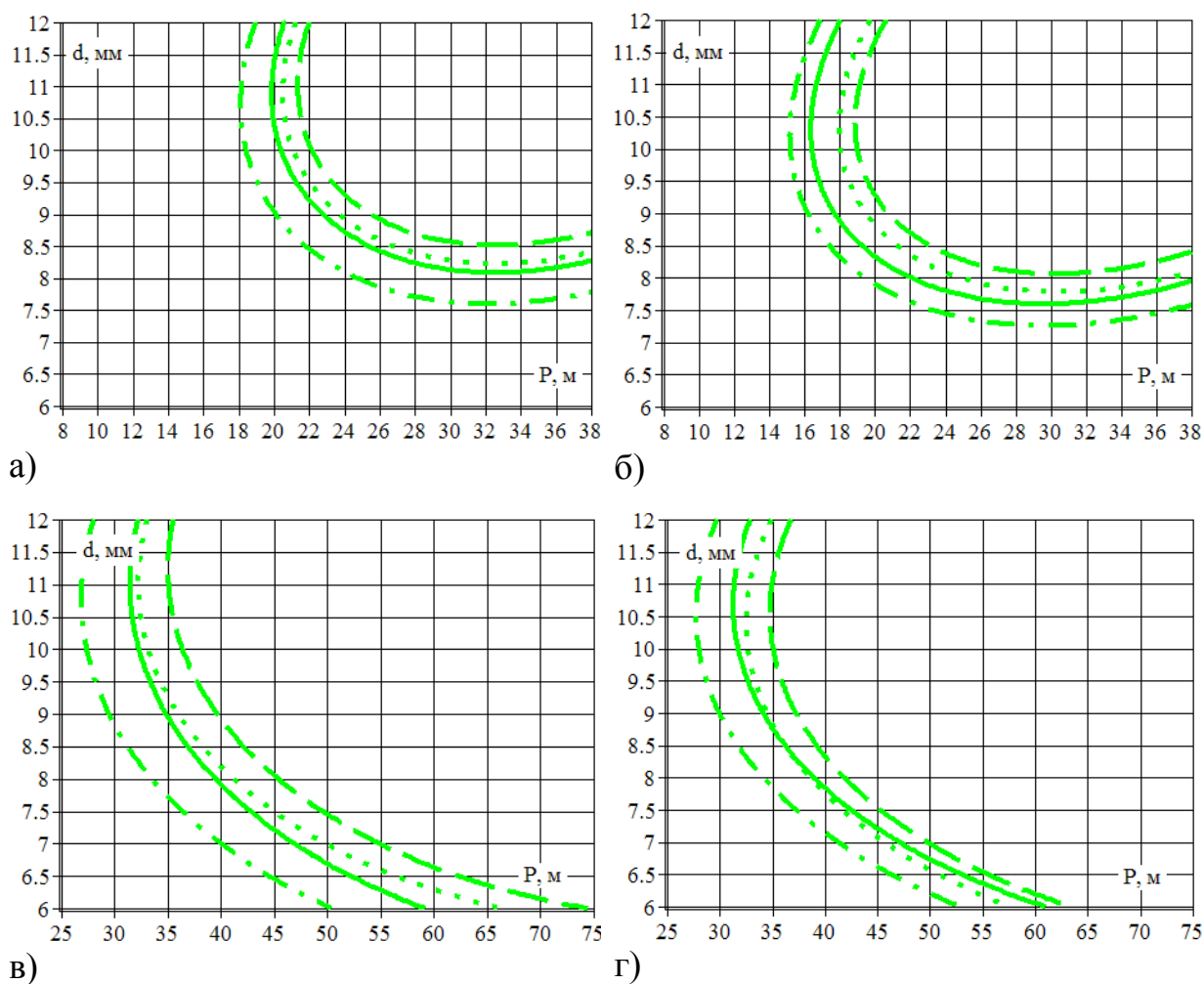
Рис. 4.7. Номограми для визначення припустимих параметрів ПКК: а) ГПВ ПЗР 33 мм; б) ГПВ НЖР 33 мм; в) ВПВ ПЗР 33 мм; г) ВПВ НЖР 33 мм;
