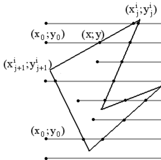
Рис. 3.9. Взаємне розтощування луча і багатокутника
