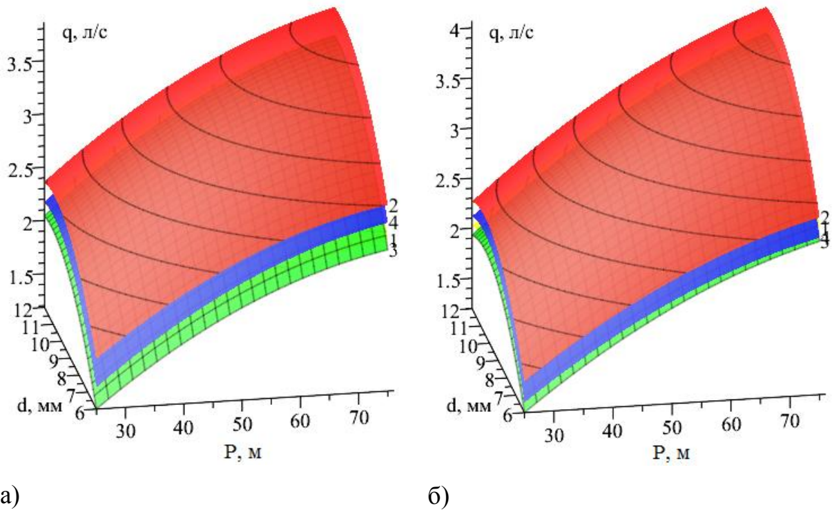
Рис. 2.11. Залежність витрат води q (л/с) від діаметра насадка d (мм) та тиску в мережі P (м) у випадку підключення до ВПВ рукава діаметром 33 мм: 1 – l=15 м, s=32 %; 2 – l=27 м, s=32 %; 3 – l=15 м, s=88 %; 4 – l=27 м, s=88 %. а) ПЗР; б) НЖР
