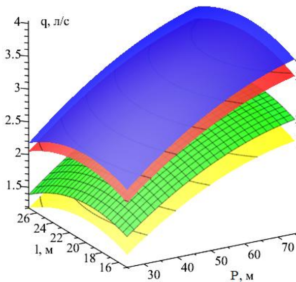
Рис. 2.8. Залежність витрат води q (л/с) від довжини рукава l (м) та тиску в мережі P (м) у разі підключення до ВПВ рукава діаметром 33 мм: 1 – s=32\% , d=6 мм; 2 – s=88\% , d=6 мм; 3 – s=32\% , d=12 мм; 4 – s=88\% , d=12 мм. а) ПЗР; б) НЖР
