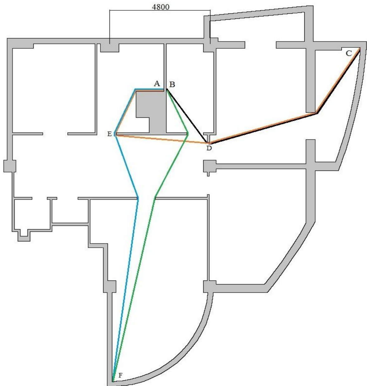
Рис. 3.11. Приклад розрахунку мінімально допустимої довжини рукава для житлового приміщення
