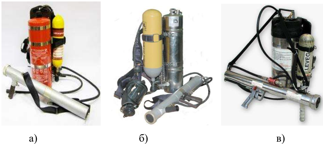
Рис. 1.14. Імпульсні ранцеві пневматичні установки пожежогасіння а) Тайфун-1-10; б) Витязь УПТ 10/1(0,4)-2; в) IFEX 3000
