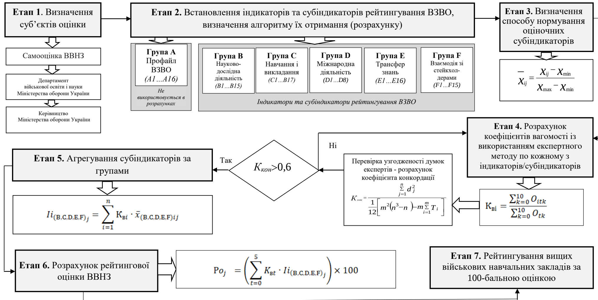
Рис. 3. Алгоритм рейтингування вищих військових навчальних закладів України
