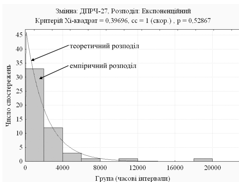
Рисунок 4.13 - Порівняння емпіричного і теоретичного розподілу інтервалів часу між надходженням викликів до ДПРЧ-27
