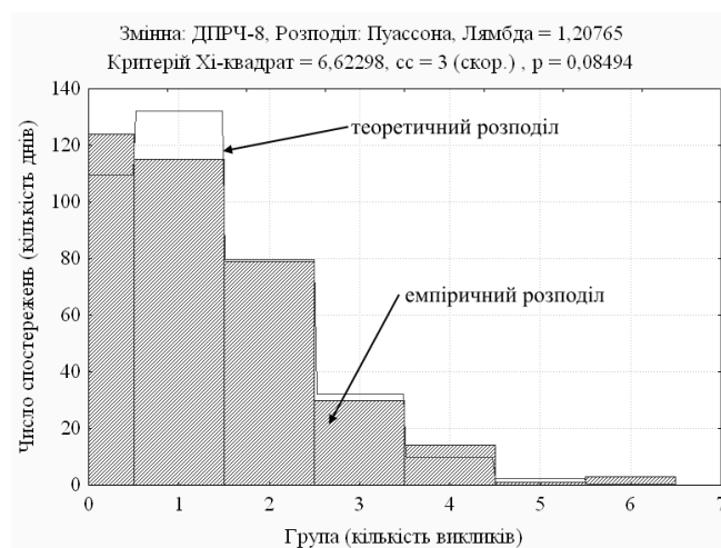
Рисунок 4.9 – Порівняння емпіричного і теоретичного розподілу кількості викликів, які надходили до ДПРЧ-8
