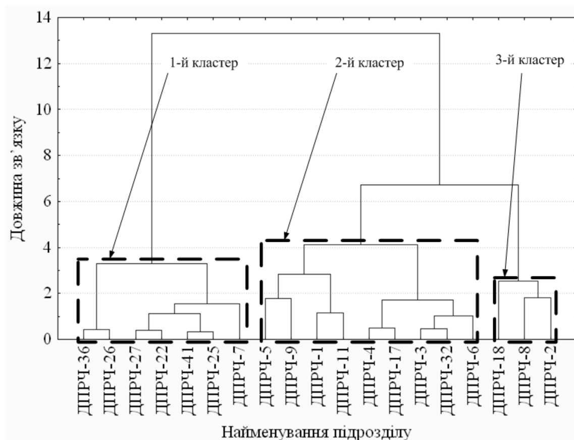
Рисунок 4.7 – Результати кластеризації (групування) АРФ за частотою викликів
