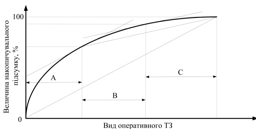
Рисунок 4.2 – Ілюстрація графічного методу визначення меж класифікаційних груп ABC на основі побудованої кумулятивної кривої
