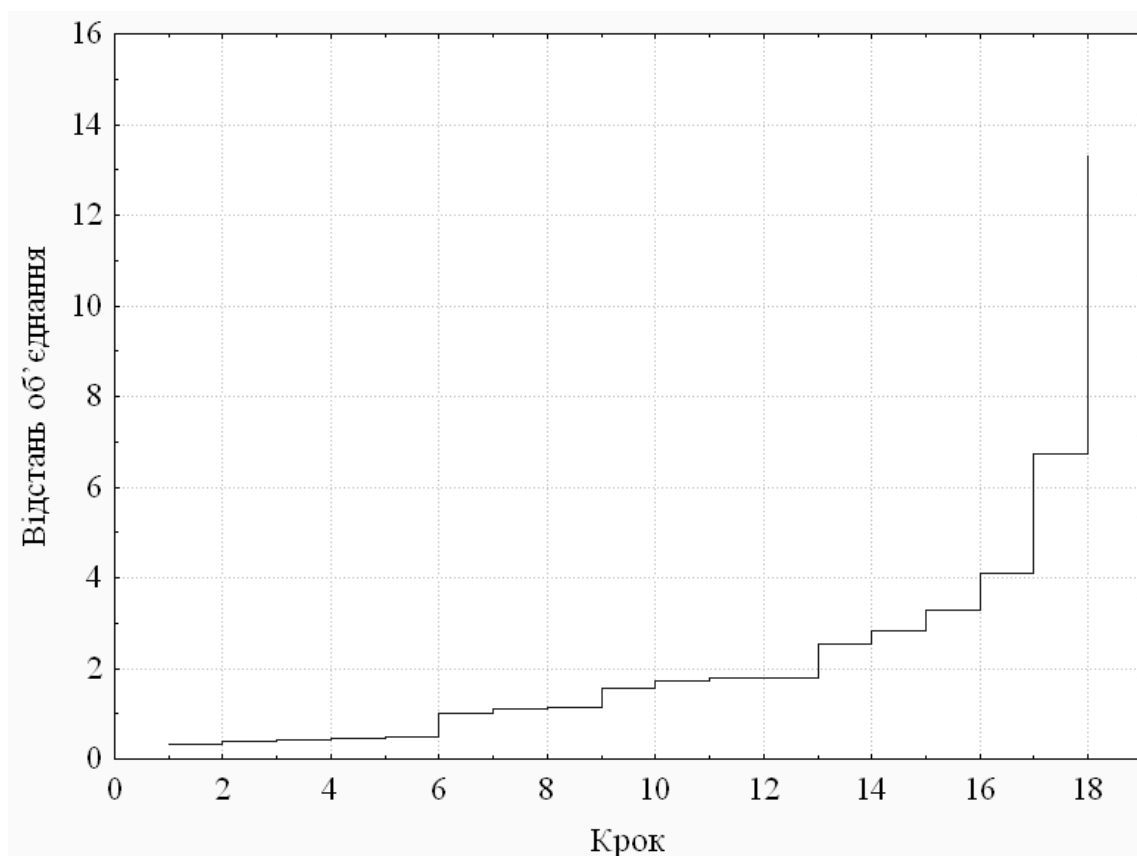
Рисунок 4.6 – Процес покрокового об'єднання змінних при проведенні ієрархічного кластерного аналізу
