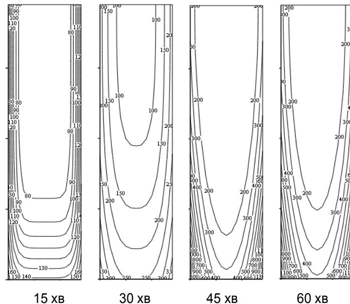
Рис. 4.15. Температурні розподіли у перерізі зразку-фрагменту дерев'яної балки з вогнезахисним просоченням ІІ типу
