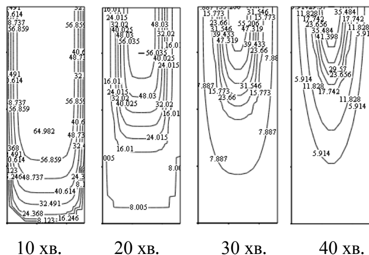
Рис. 5.16. Розподіл значень міцності (МПа) на стискання для розподілу температур, визначених експериментально, у дерев'яній балці з вогнезахисним просоченням I типу з врахуванням зони обвуглювання
