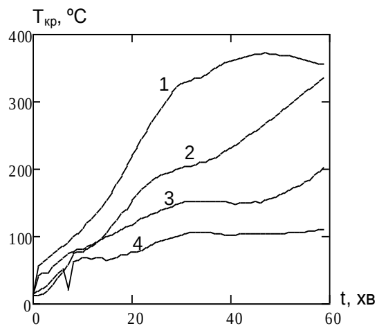
Рис. 4.17. Залежності критичної температури обвуглювання від часу випробування: 1 – без вогнезахисту; 2 – вогнезахисне просочення I типу; 3 – вогнезахисне просочення II типу; 4 – вогнезахисне просочення III типу
