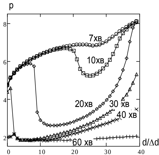
Рис. 4.10. Залежності показника ступеня рівняння від параметру d для різних моментів часу дії пожежі
