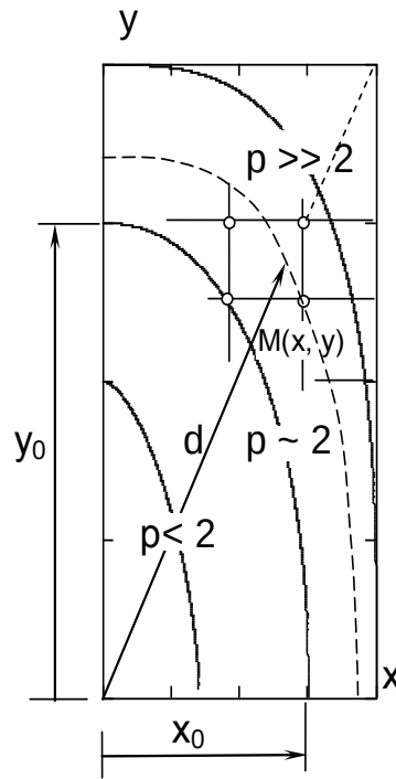
Рис. 4.9. Схема апроксимації ізотерм в перерізі фрагмента дерев'яної балки
