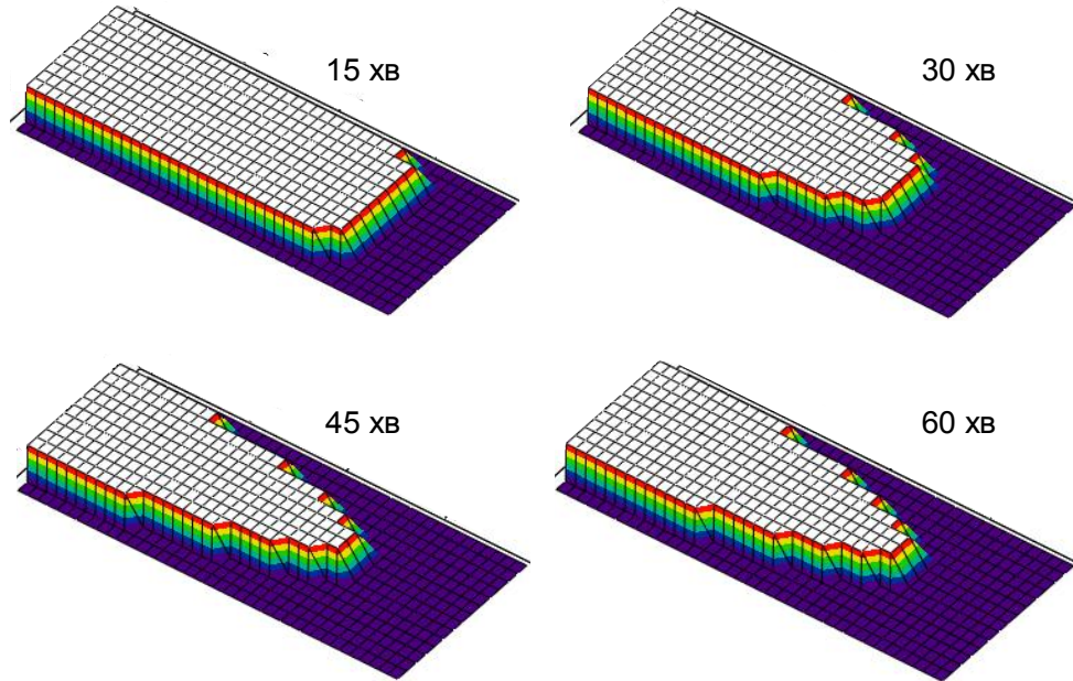
Рис. 4.20. Динаміка зміни обвугленої зони фрагменту із вогнезахисним просоченням II типу
