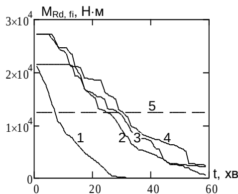
Рис. 5.19. Залежності максимального моменту від часу вогневого впливу пожежі з врахуванням зони обуглювання: 1 – дерев'яної балки із експериментальними температурними розподілами; 2 – дерев'яної балки із вогнезахисним просоченням I типу; 3 – дерев'яної балки із вогнезахисним просоченням II типу; 4 – дерев'яної балки із вогнезахисним просоченням III типу; 5 – діючий момент у небезпечному перерізі балки
