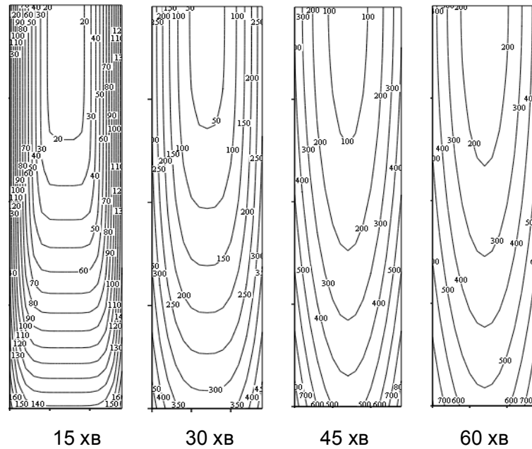
Рис. 4.14. Температурні розподіли у перерізі зразку-фрагменту дерев'яної балки з вогнезахисним просоченням І типу
