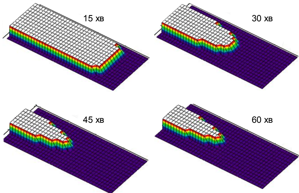
Рис. 4.21. Динаміка зміни обвугленої зони фрагменту із вогнезахисним просоченням III типу.
