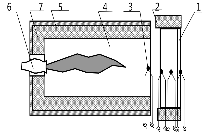
Рис. 2.2. Експериментальна установка для вогневих випробувань зразків-фрагментів дерев'яних балок: 1 – зразок для дослідження, 2 – теплоізоляція зразка; 3 – місця установки термопар; 4 – камера теплового впливу печі; 5 – корпус печі; 6 – газовий пальник; 7 – теплоізоляція камери теплового впливу печі
