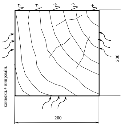
Рис. 5.20. Розрахункова схема перерізу дерев'яної балки для відпрацювання процедур запропонованого метода розрахункової оцінки вогнестійкості
