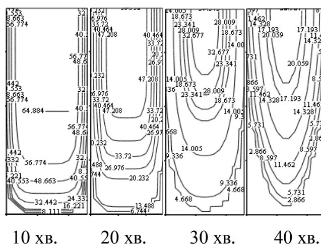
Рис. 5.18. Розподіл значень міцності (МПа) на стискання для розподілення температур, визначених експериментально, у дерев'яній балці з вогнезахисним просоченням III типу з врахуванням зони обвуглювання
