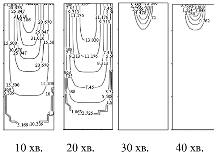
Рис. 5.15. Розподіл значень міцності (МПа) на стискання для розподілу температур, визначених експериментально, у дерев'яній балці без просочення з врахуванням зони обвуглювання
