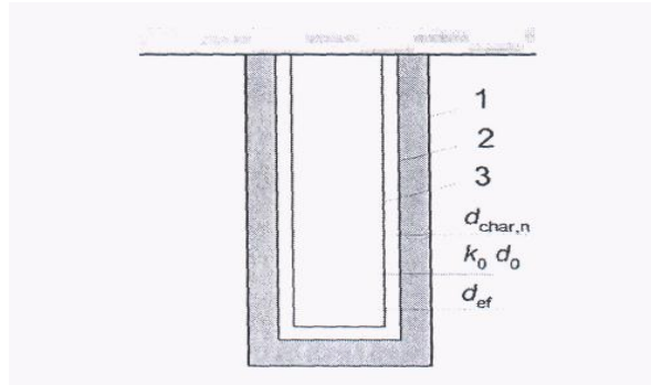
Рис. 1.2. Визначення залишкового і ефективного (робочого) поперечного перерізу: 1 – початкова поверхня елемента; 2 – межа площі залишкового перерізу; 3 – межа площі ефективного (робочого) перерізу
