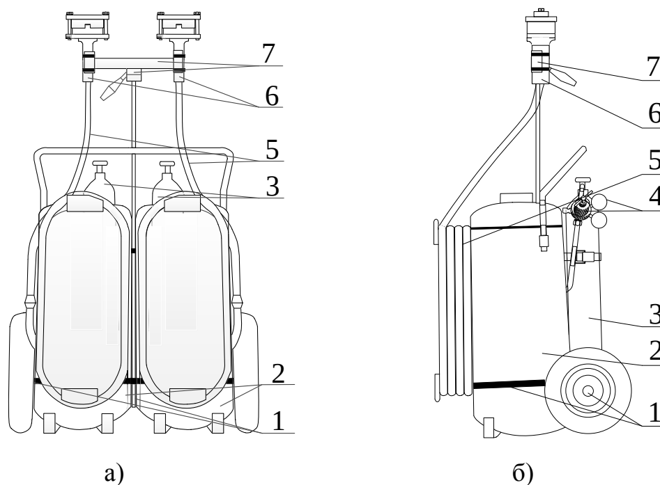
Рис. 2.1 Дослідна установка АУГГУС-М: а) фронтальна проекція; б) профільна проекція;
