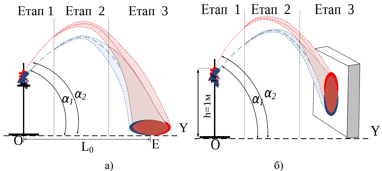
Рис. 2.13 Схеми подачі на осередок пожежі двох незалежних один від одного розпиленних струменів бінарного потоку ГУС стволами-розпилювачами, націленими в епіцентр горіння за незалежними траєкторіям руху при гасінні:
