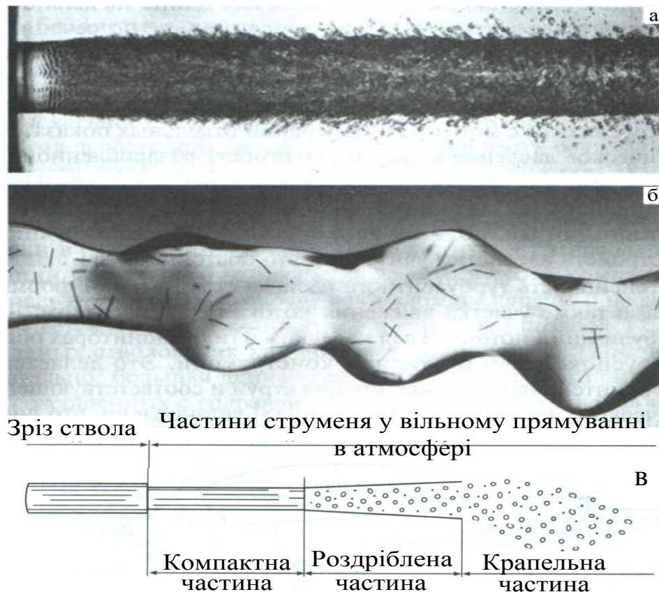
Рис. 1.3 Трансформація водяного струменя: а) фото компактної частини струменя; б) фото роздрібненої частини струменя; в) схематичне уявлення руху незатоплюваного струменя в повітрі
