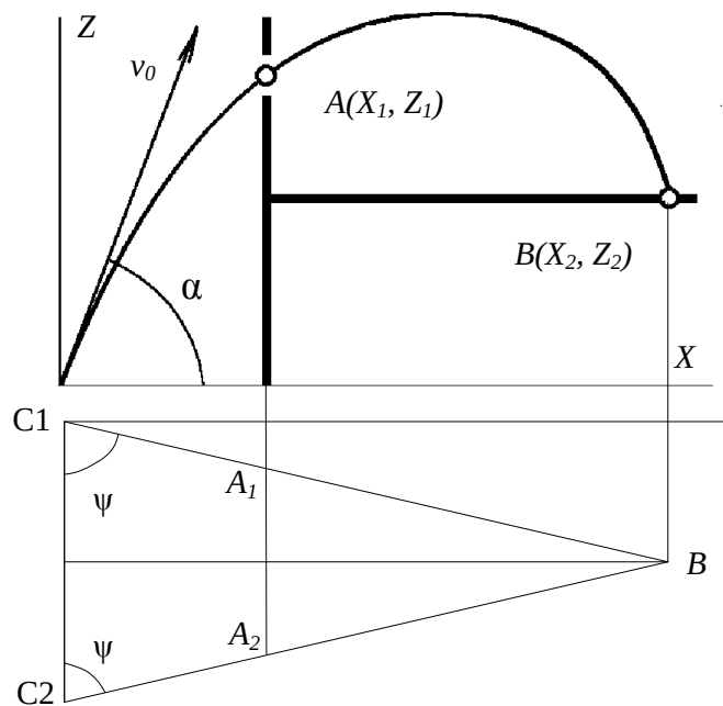
Рис. 2.8 Фронтальна і горизонтальна проекції щодо визначення двох симетричних осьових траєкторій руху компонент ГУС для обох струменів що охоплюють задані точки A і B
