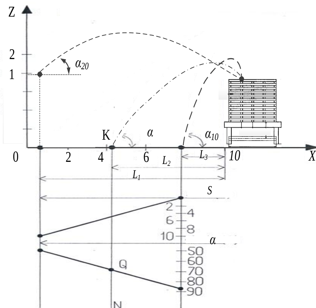
Рис. 4.2 Введення обмежень і номограма до задачі 4 – подача потоку ВГР/ГУС в точку на рівень поверхні модельного вогнища 1А
