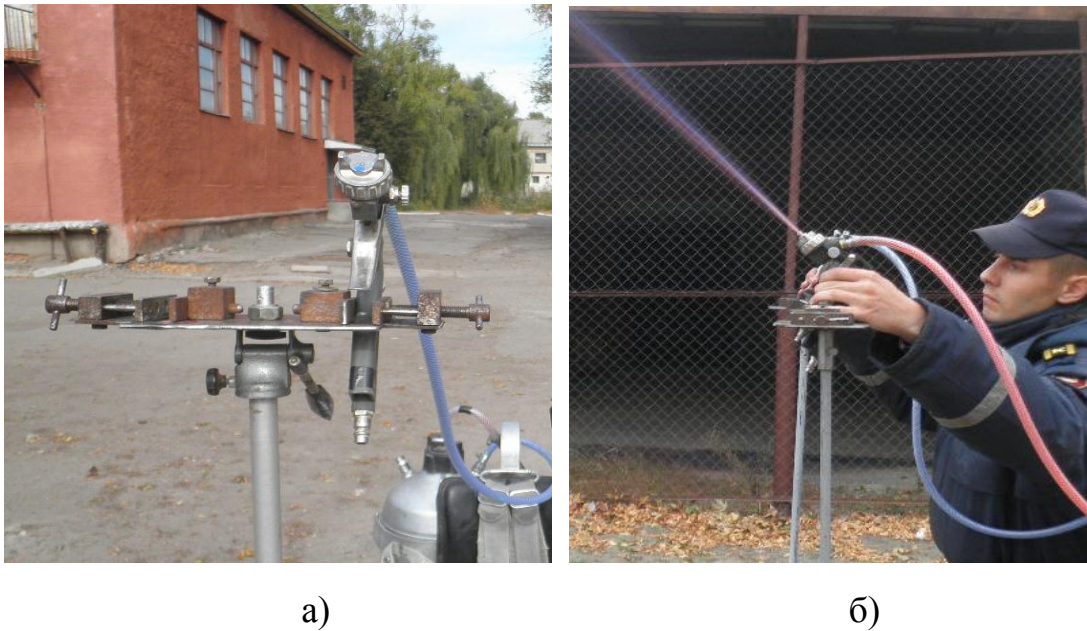
Рис. 3.2 Пристрій для фіксації кутів нахилу до горизонту і кутів відхилення стволів-розпилювачів: а) фіксація одного зі стволів-розпилювачів під заданим кутом нахилу \alpha_1 (вид з боку вихідного отвору); б) задіяння закріпленого у допоміжному пристрої ствола-розпилювача при \alpha_1 = 45^\circ (вид збоку)
