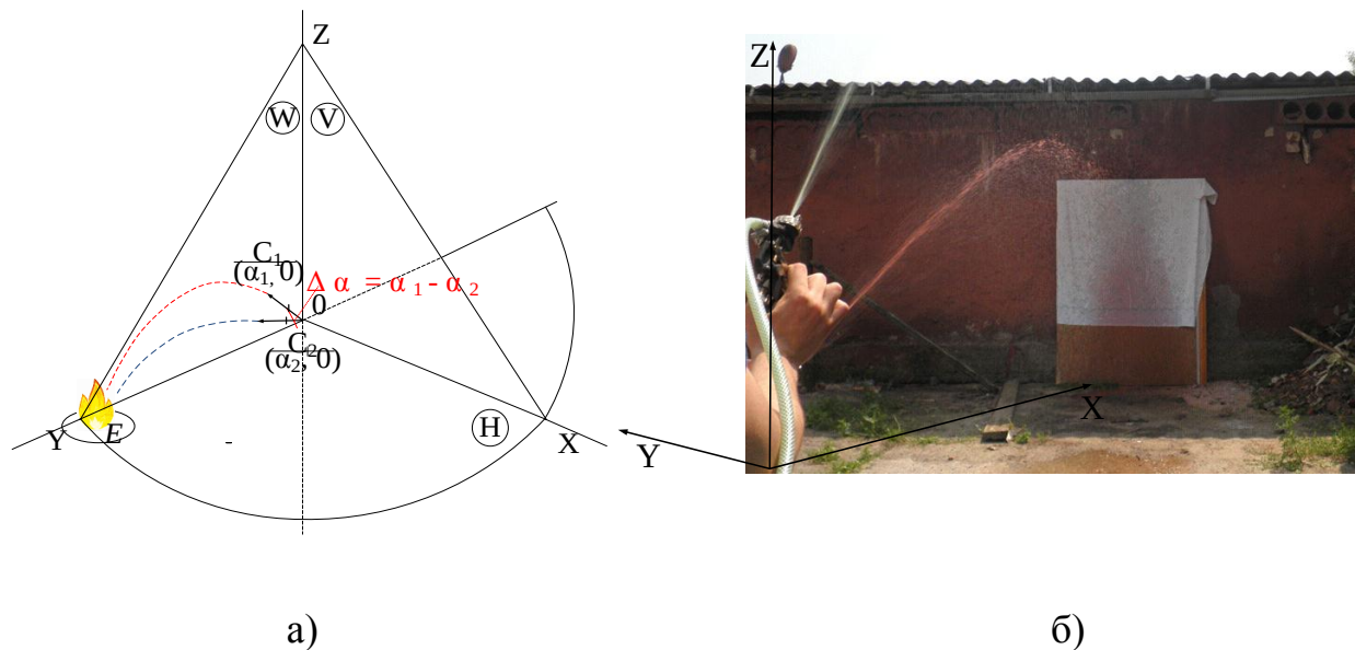
Рис. 2.14 Подача струменів на пожежогасіння: а) схема розташування стволів-розпилювачів C1 і C2, що подають в епіцентр пожежі (точка E) компоненти бінарного потоку ГУС, \alpha_1 > \alpha_2 – кути нахилу стволів до горизонту, \psi_1 = \psi_2 = 0 – кути відхилення; б) фото подачі компонент розпиленої води з однієї точки установкою АУГГУС двома струменями ( \alpha_1 > \alpha_2 ; \psi_1 = \psi_2 = 0 )
