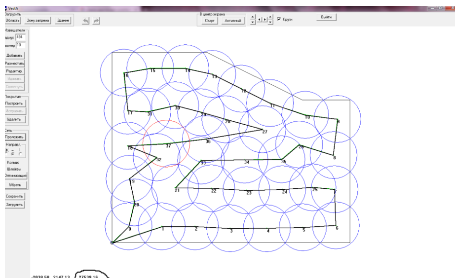
Рис. 3. Пример розв'язання задачі формування шлейфів пожежної сигналізації з переважною горизонтальною орієнтацією
