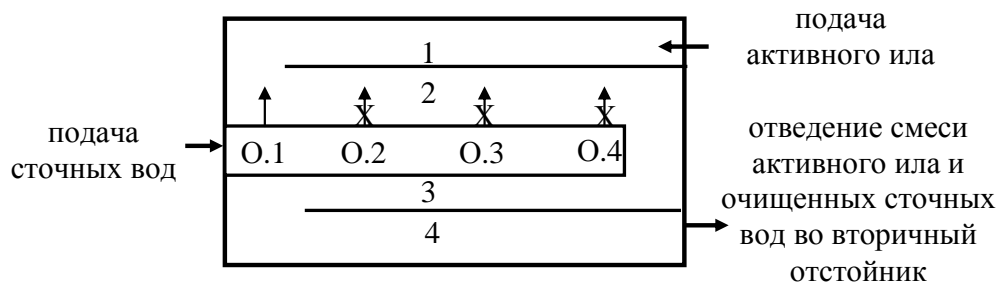
Рис. 1. Схема секции аэротенка: 1 – первый коридор, 2 – второй коридор, 3 – третий коридор, 4 – четвертый коридор аэротенка; О.1, О.2, О.3, О.4 – впускные окна
