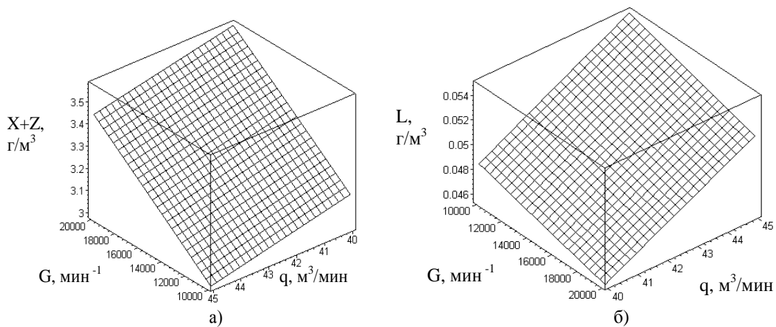
Рис. 3. Изменение концентраций во 2-м коридоре в зависимости от расхода сточных вод ( q ) и градиента скорости в турбулентном потоке ( G ): а) активного ила ( X+Z ); б) концентрации загрязнений ( L )
