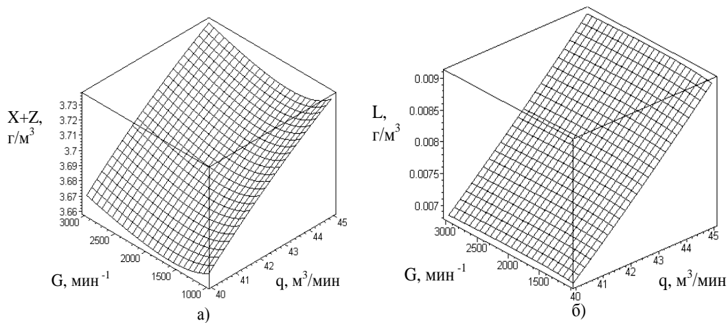
Рис. 4. Изменение концентраций в 3-4 коридорах в зависимости от расхода сточных вод ( q ) и градиента скорости в турбулентном потоке ( G ): а) активного ила ( X+Z ); б) концентрации загрязнений ( L )
