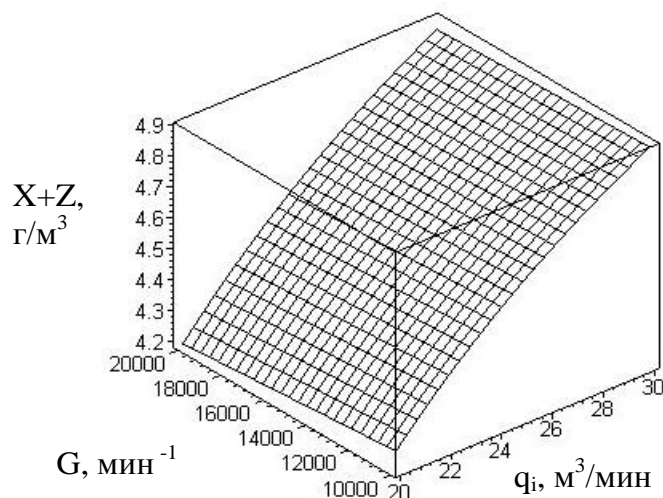
Рис. 2. Изменение концентрации активного ила ( X+Z ) в 1 коридоре аэротенка в зависимости от его расхода ( q_i ) и градиента скорости в турбулентном потоке ( G )
