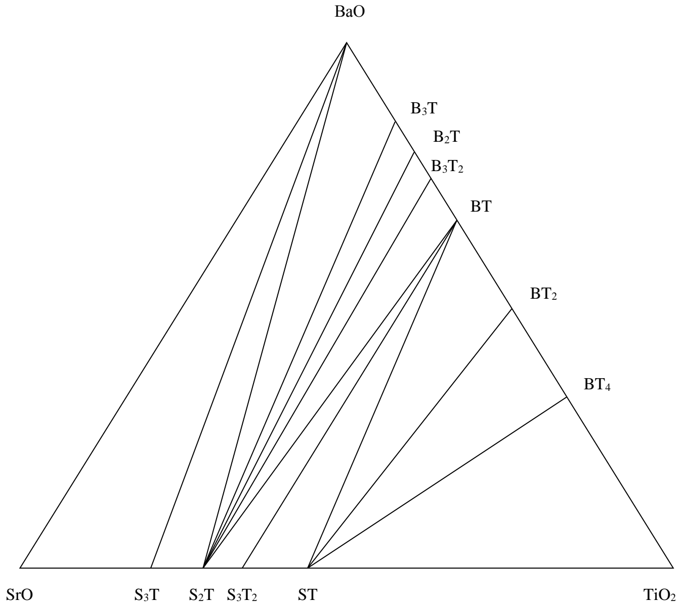
Рисунок 1 – Триангуляція системи \text{BaO} - \text{SrO} - \text{TiO}_2 при 1380^\circ\text{C} (B – \text{BaO} ; S – \text{SrO} ; T – \text{TiO}_2 ).
