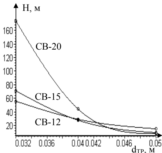
Рис. 3 – График зависимости напора в точке ввода от диаметра трубопровода ряда РС
