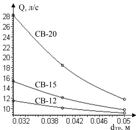
Рис. 1 – График зависимости расхода жидкого ОВ в точке ввода от диаметра трубопровода ряда РС
