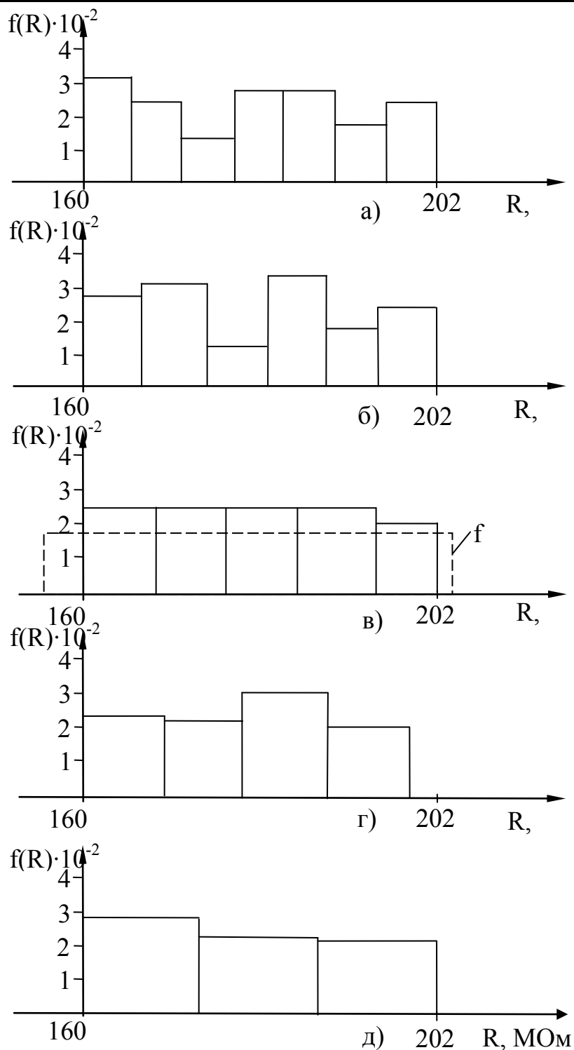
Рис. 1. Гистограмма распределения значений сопротивления изоляции при различных способах разбиения вариационного ряда
