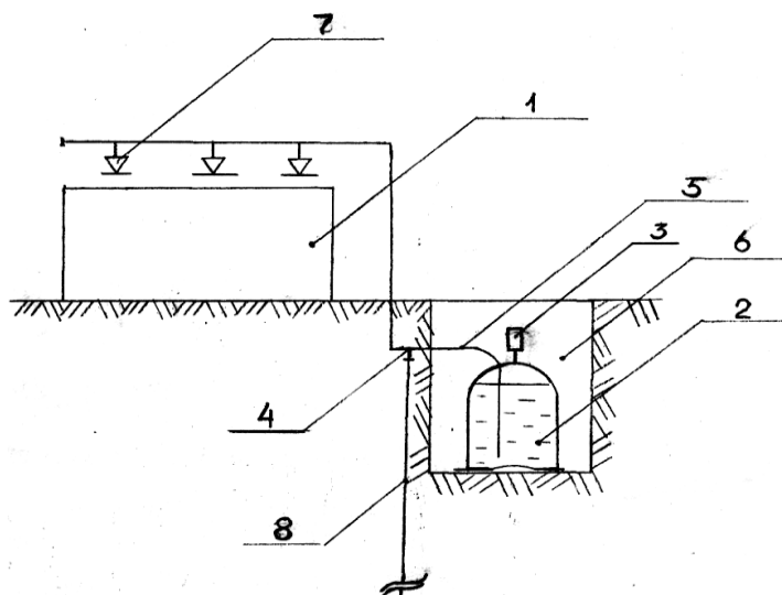
Рис. 1. Принципова схема дренчерної установки пожежегасіння з пороховим акумулятором тиску: 1 – штабель боєприпасів; 2 – резервуар з водою; 3 – пороховий акумулятор тиску; 4 – розподільчий клапан; 5 – трубопровід дренчерної системи пожежегасіння; 6 – захисна споруда; 7 – дренчер; 8 – трубопровід з насосної станції
