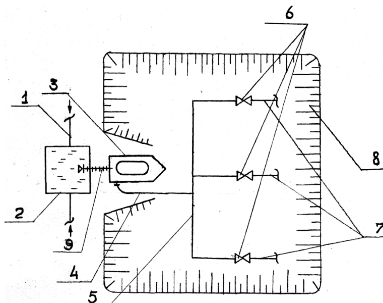
Рис. 2. Схема захисного капоніру: 1 – з'єднувальні трубопроводи з сусідніми водоймами; 2 – водойма; 3 – стаціонарна насосна установка (пересувна пожежна техніка); 4 – трубопровід підключення (пожежний рукав); 5 – розподільчий трубопровід (колектор); 6 – вентилі розподільчого вузла; 7 – трубопровід до дренчерної системи; 8 – захисний капонір
